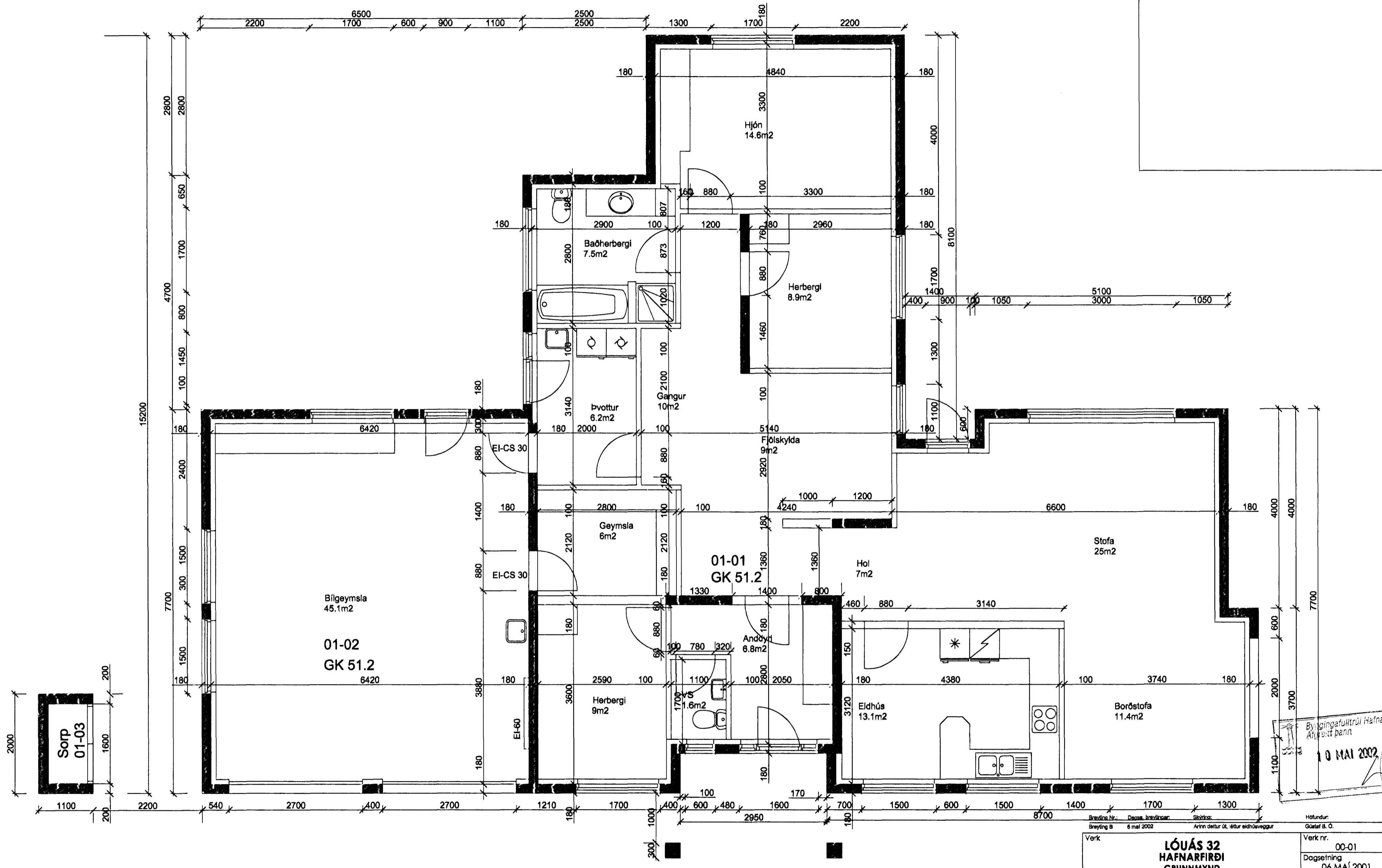
GRUNNMYND MKV. 1:50
