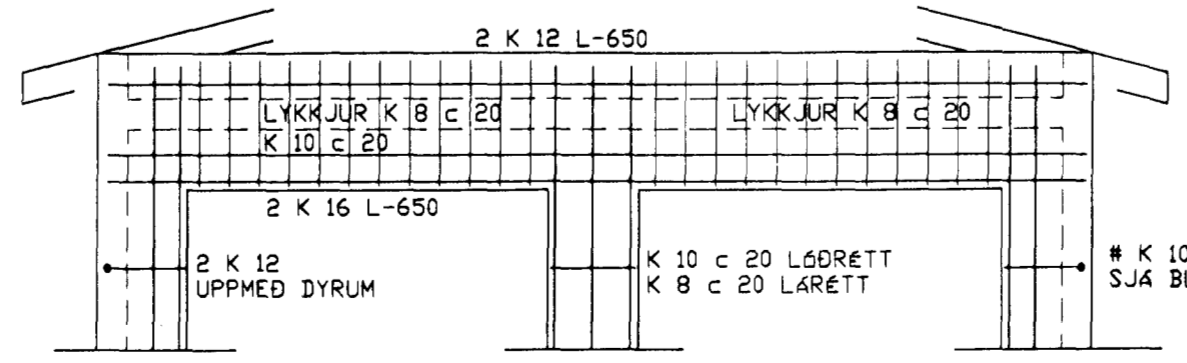
B-1 1:50
