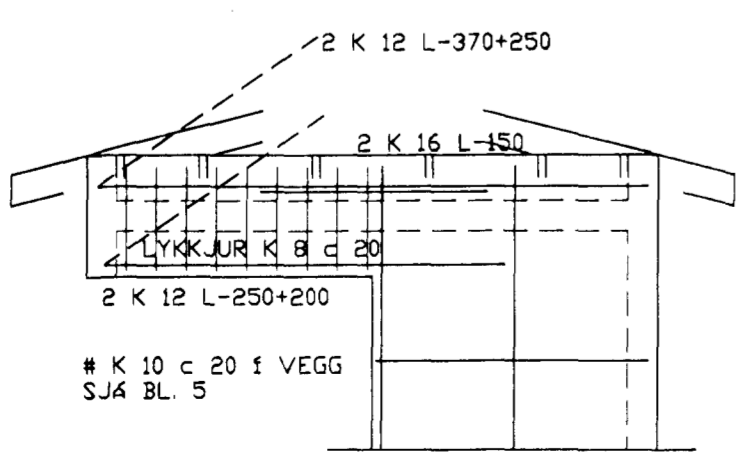
B-2 1:50
