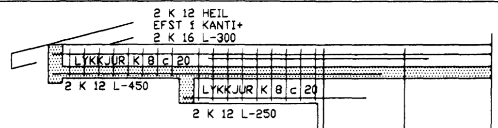
B-3 1:50
