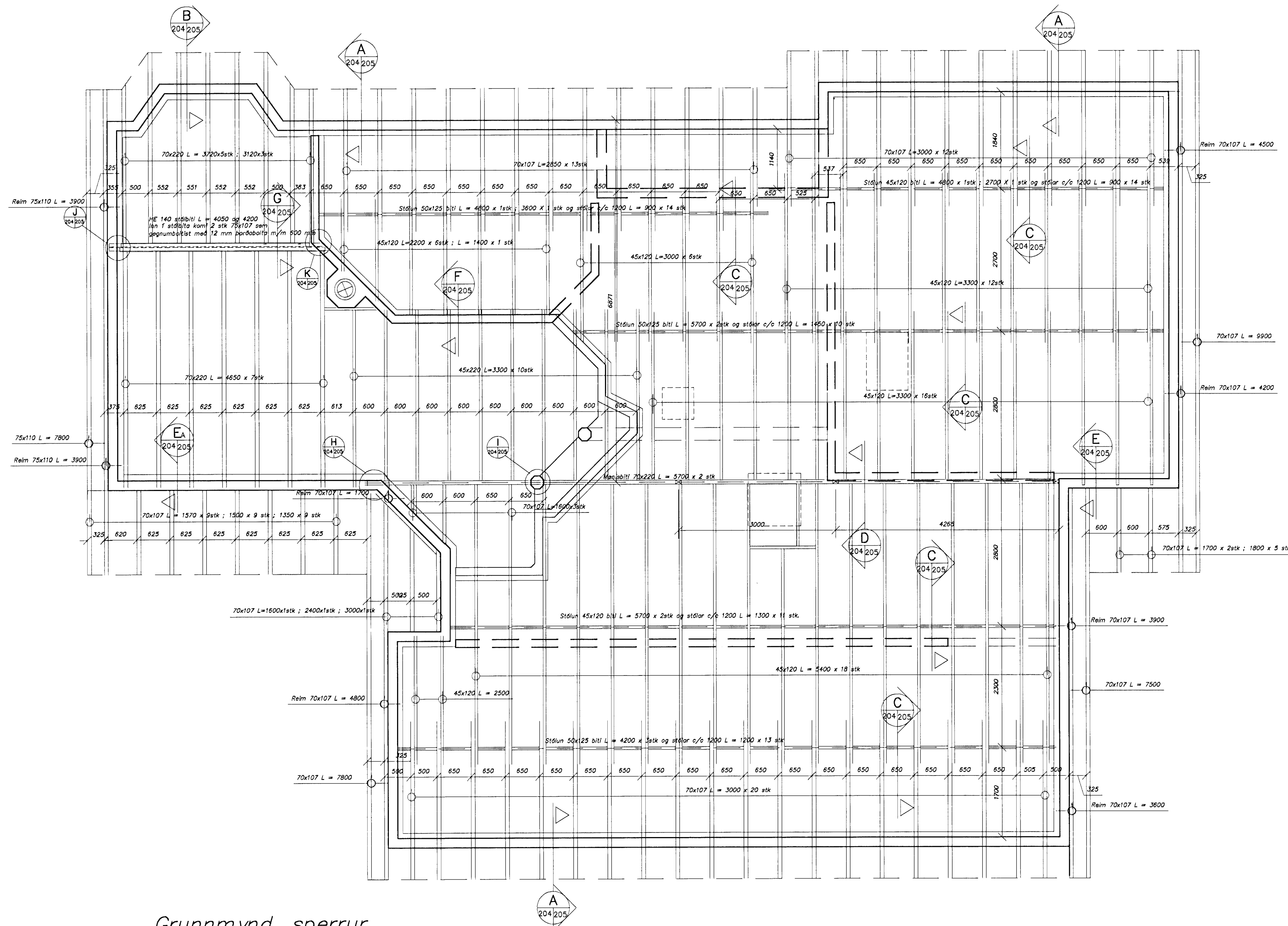
Grunnmynd, sperrur Mælikvarði 1:50
