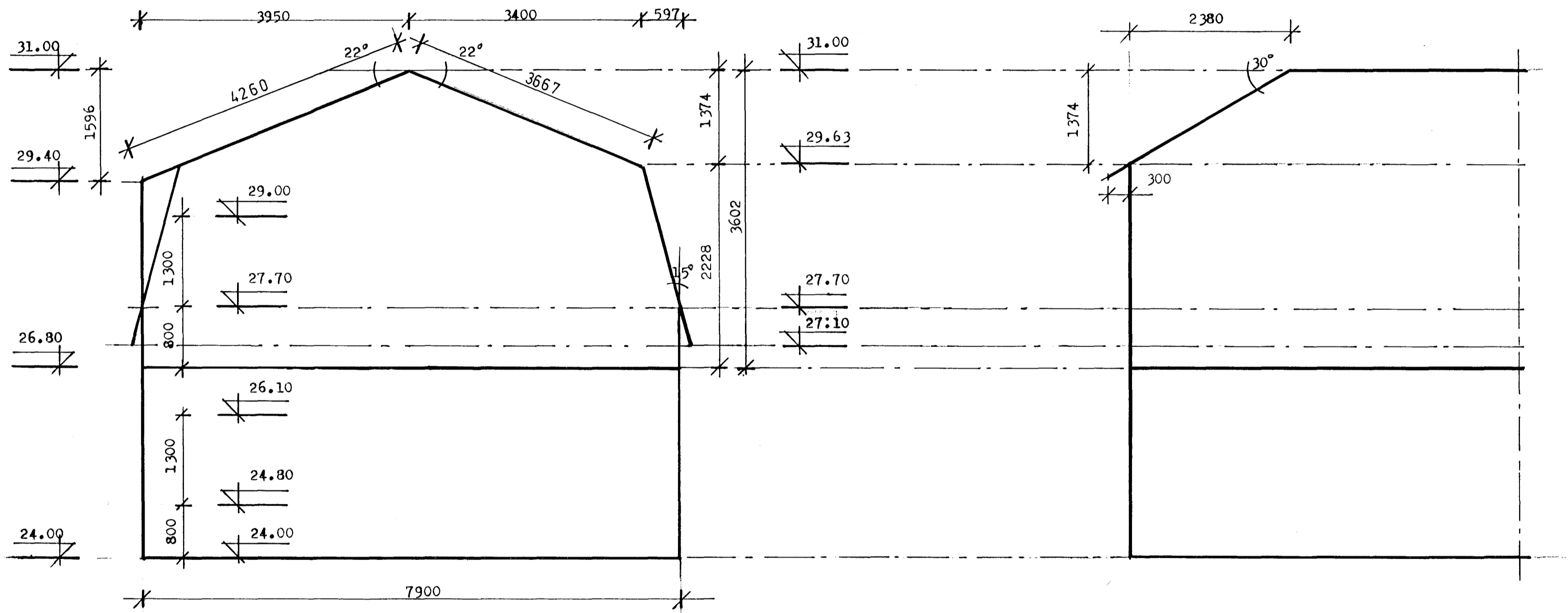
snið A - A kerfismynd.
