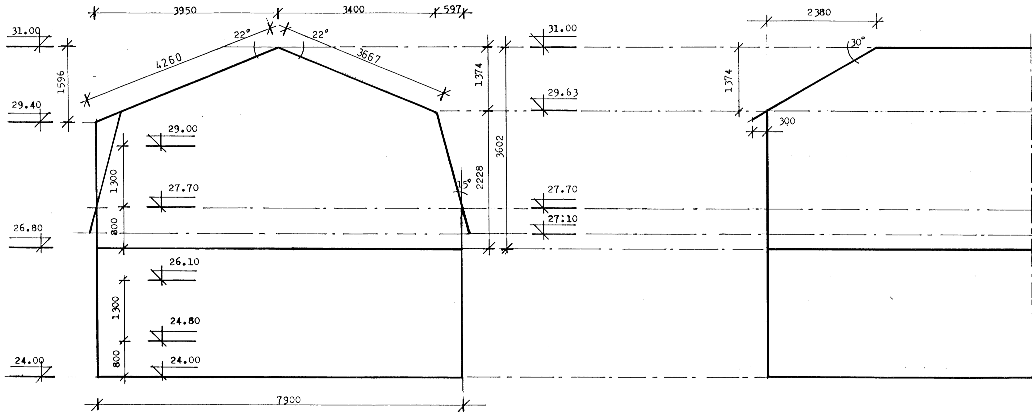
langsnið C - C kerfismynd.
