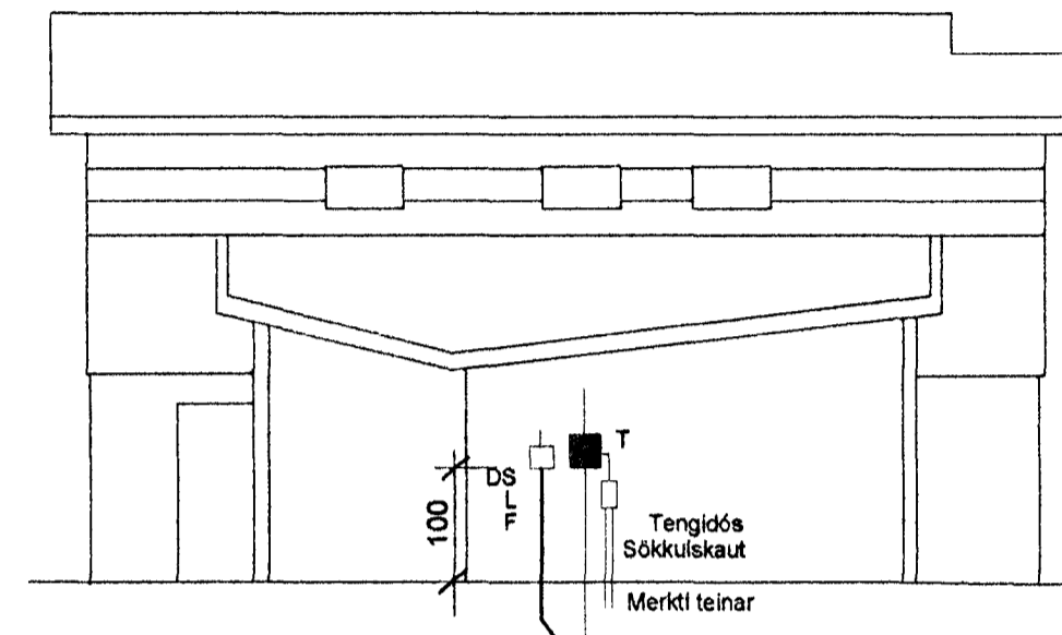
Snið a-a mkv. 1:100
