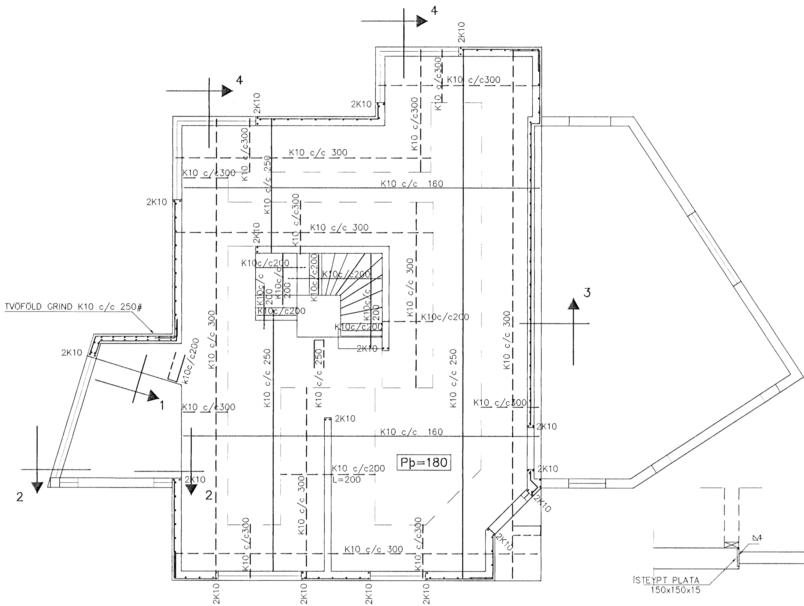
GRUNNMYND 1:50
