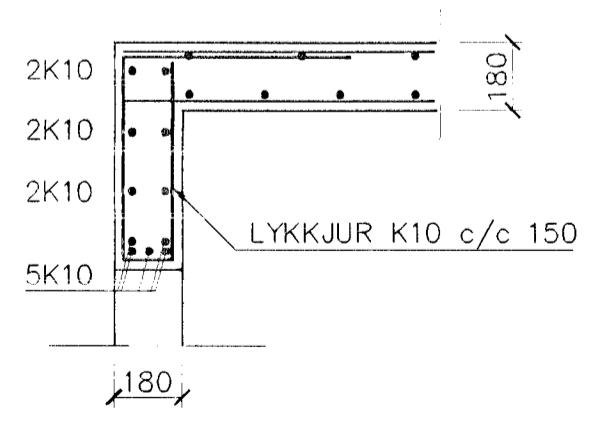
SNID 4 1:20
