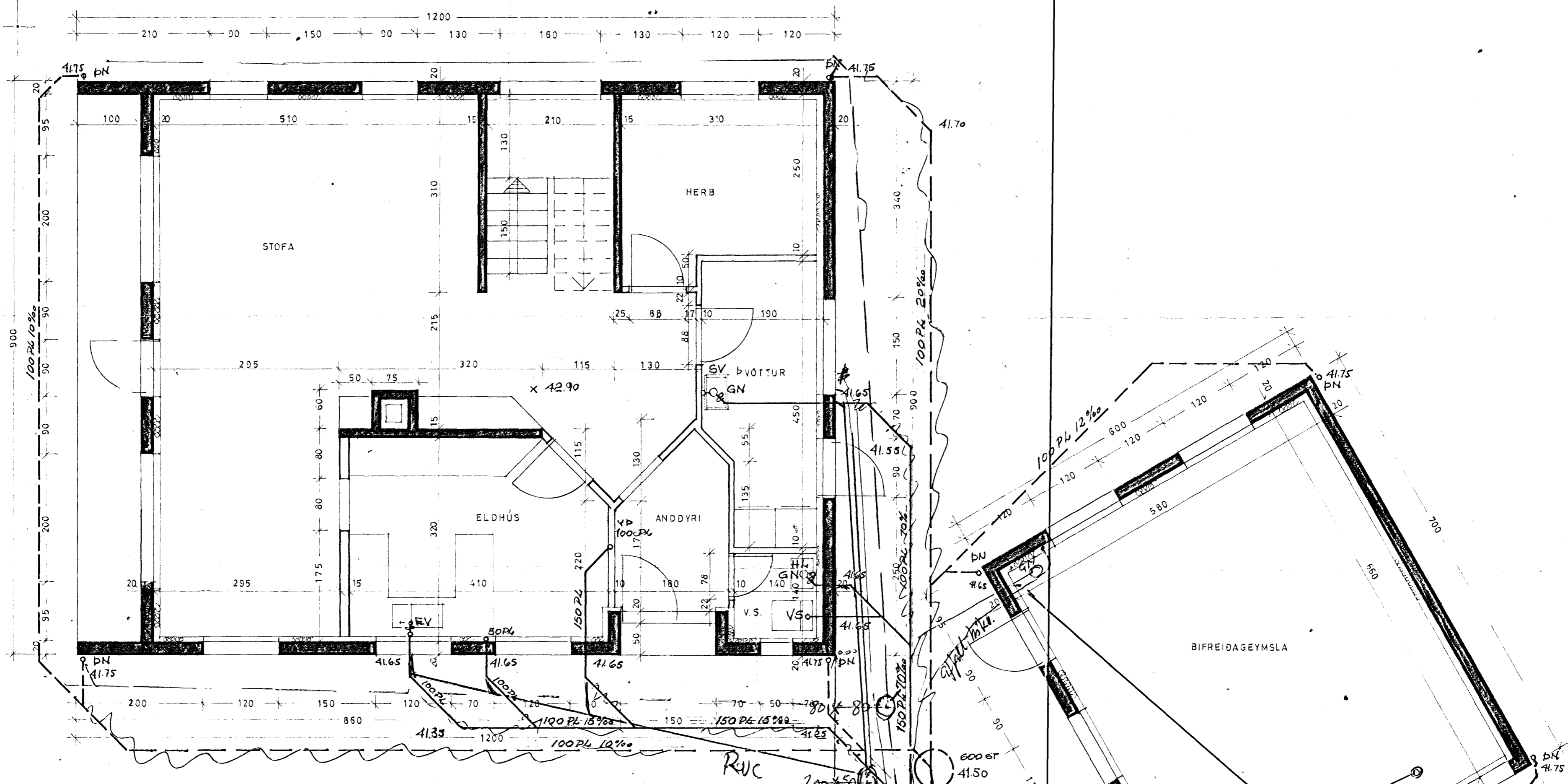
GRUNNMÝND 1:50 FRÆBENNSLI
