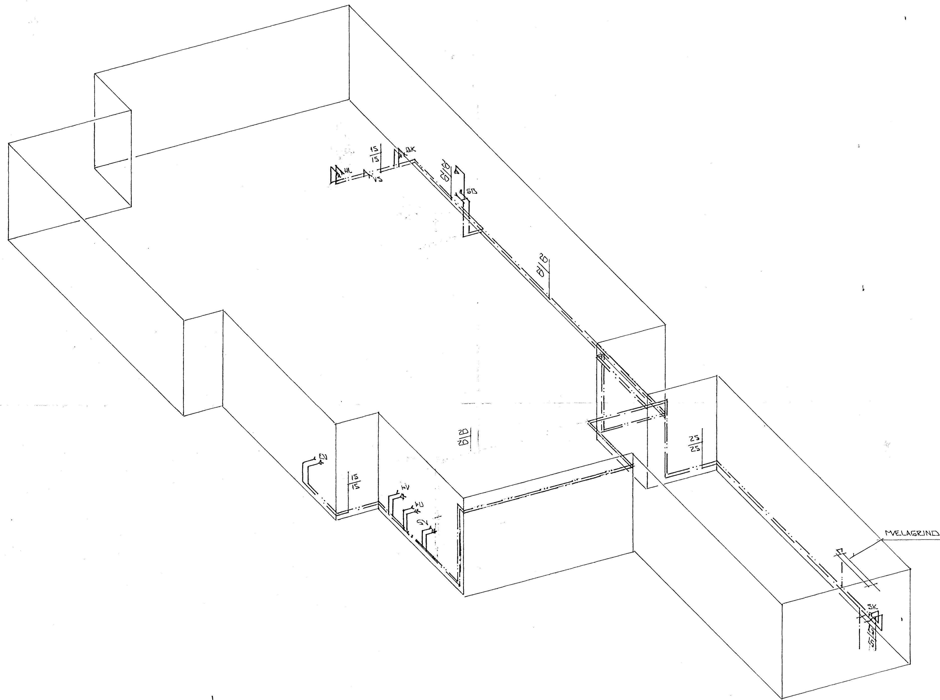
RÚMMYND VATNSLAGNA 1:50 1505 B
