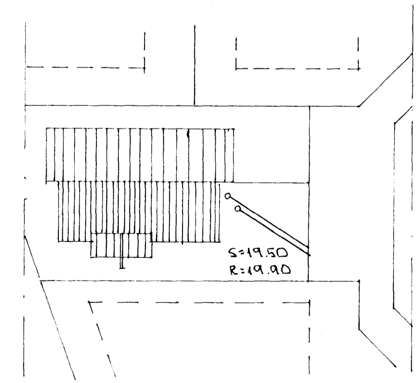
AFSTÖÐUMYND \times 1:500
