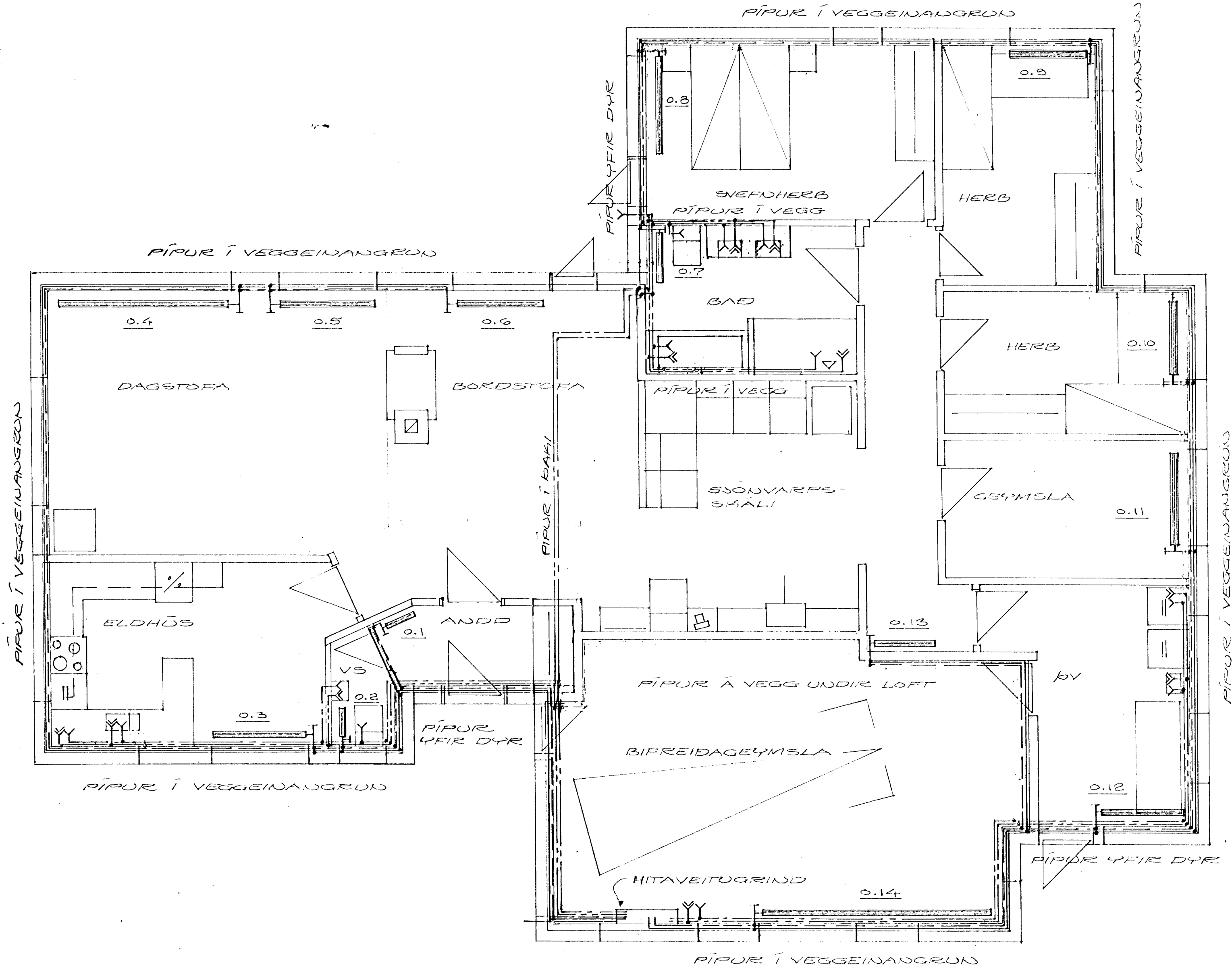
GRUNNMYND, M=1:50
