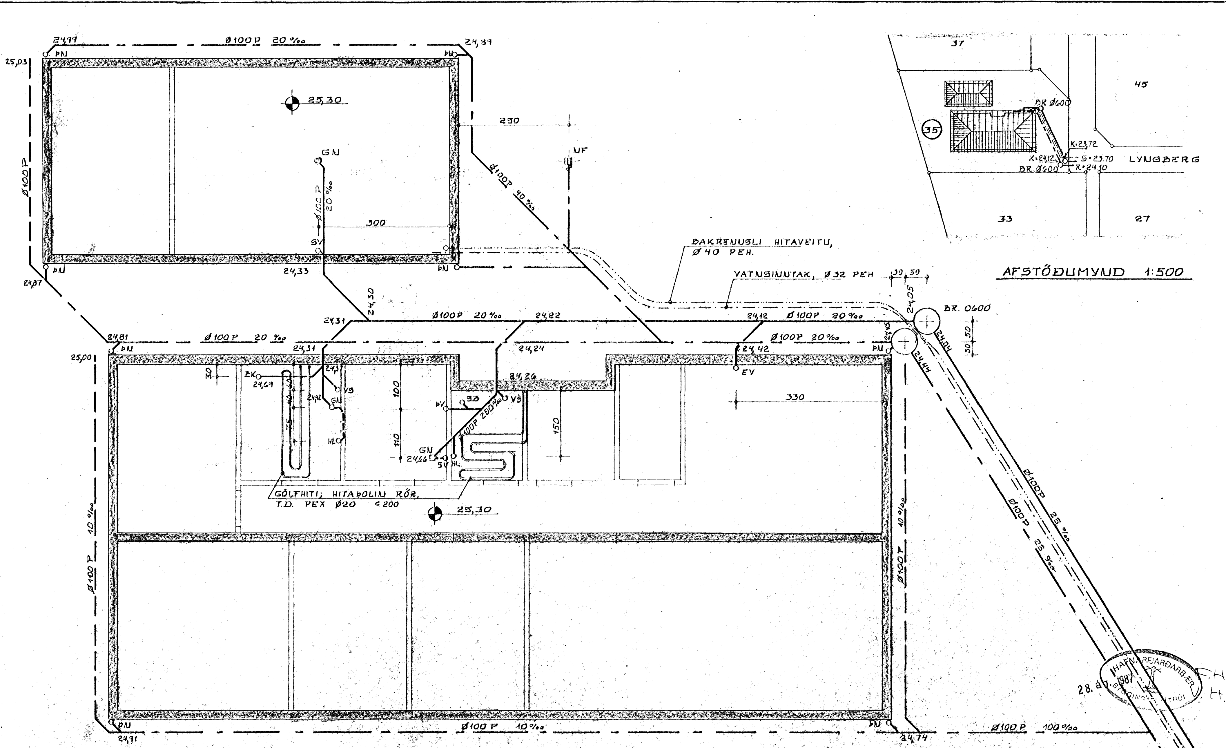
GRUNNMYND 1:50
