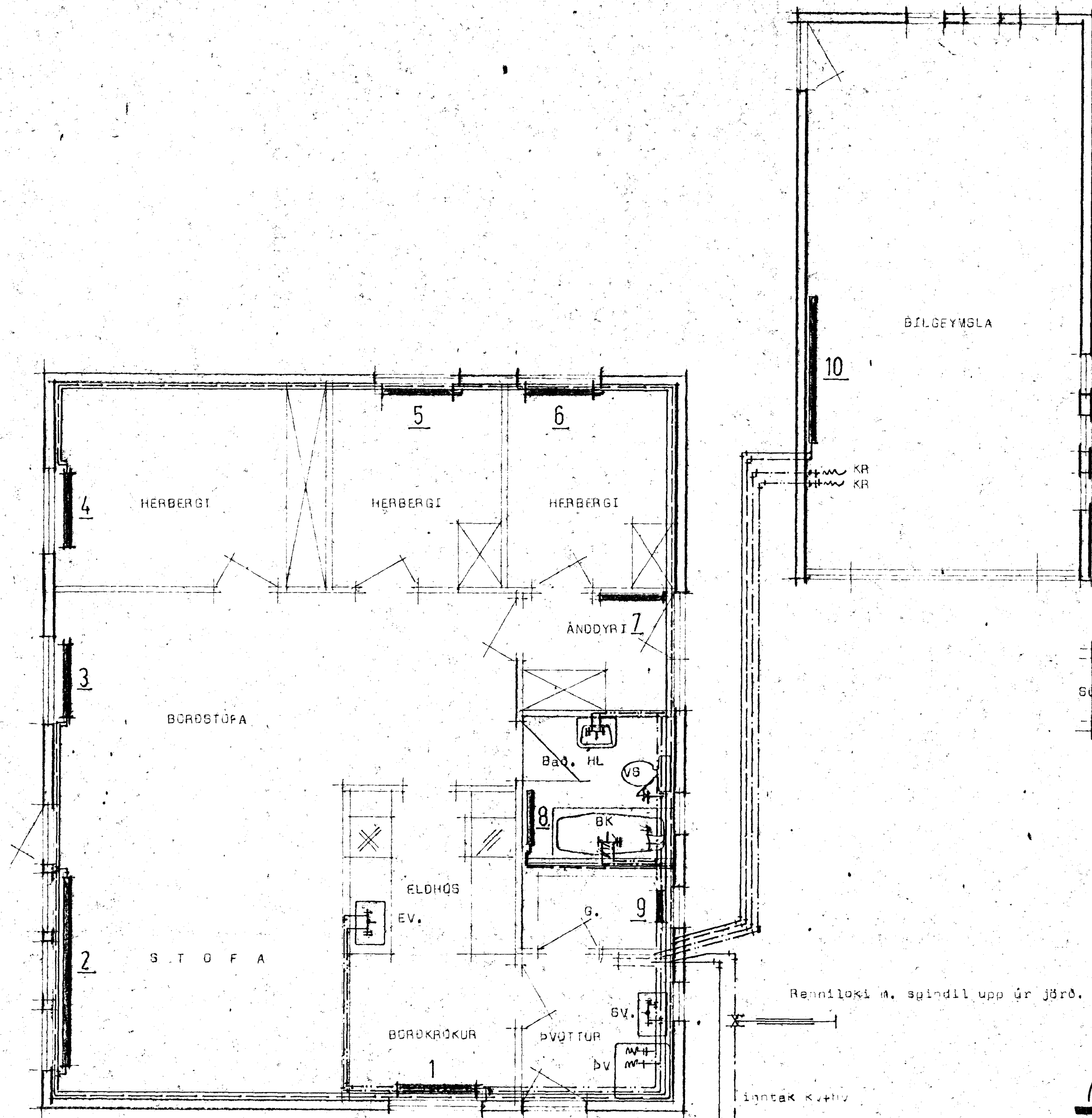
Grunnmynd Mk 1:50
