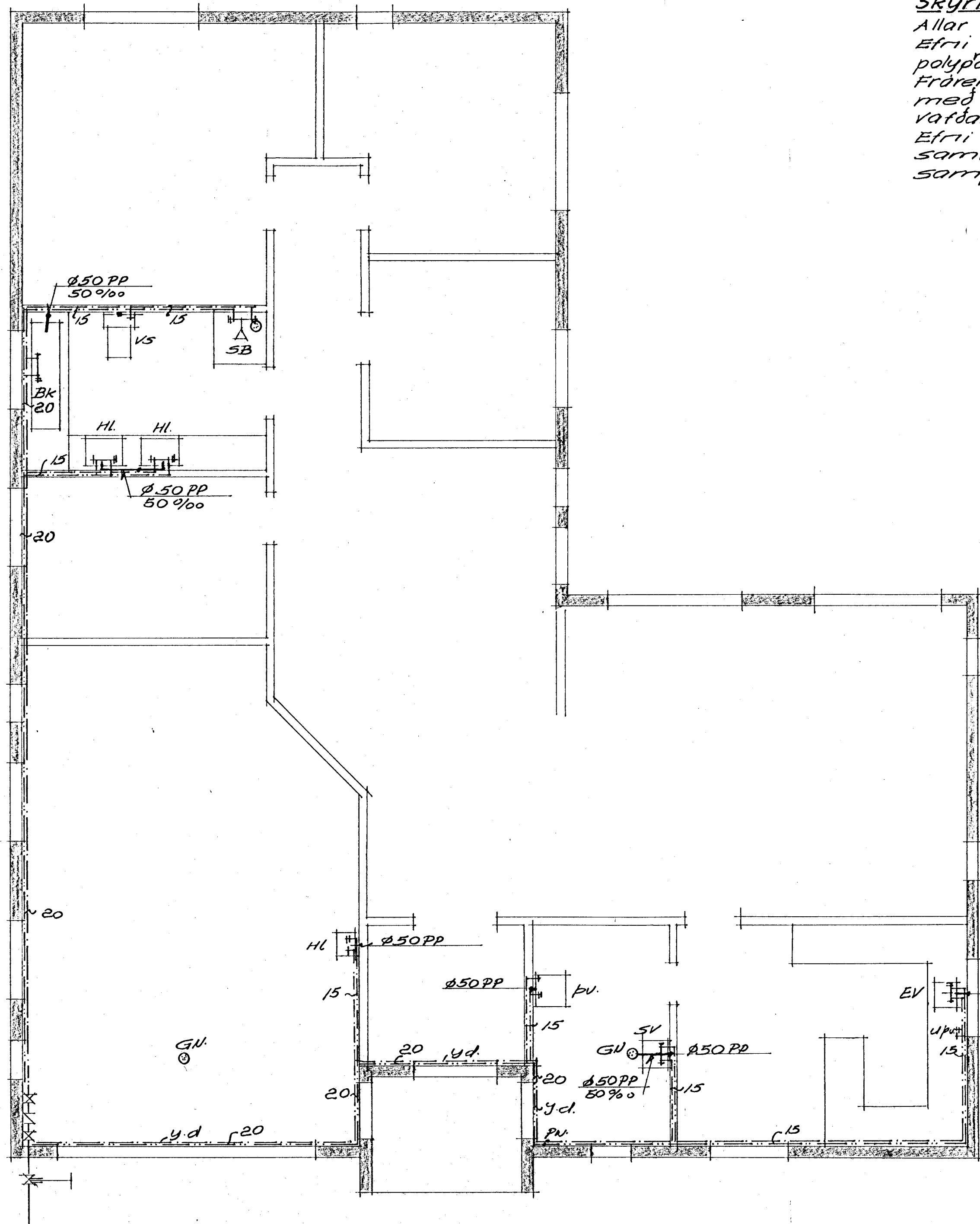
Grunnmynd M:50 Vatns- og frárennslislagnir
