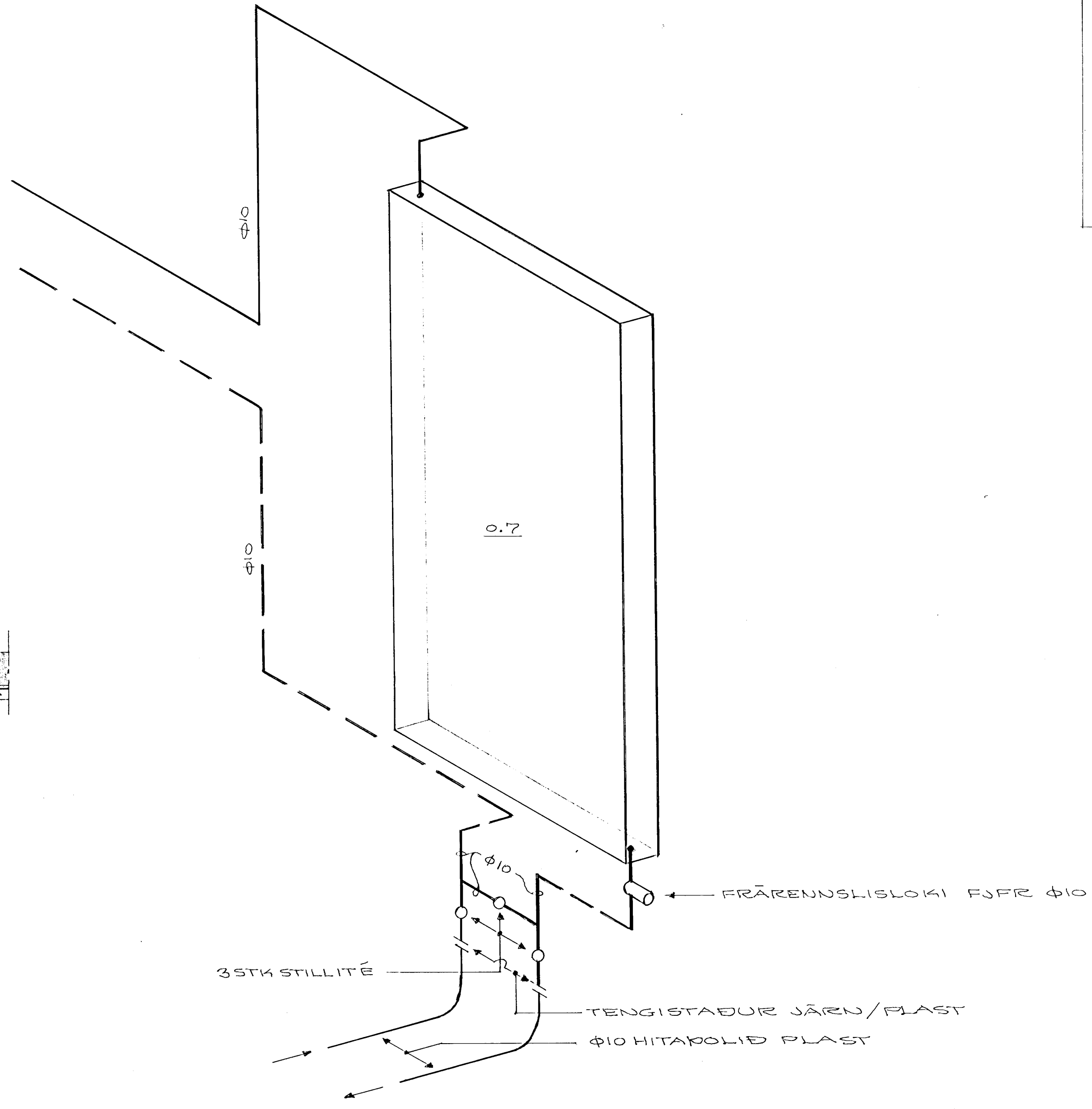
TENGING OFNFRÄRENNSLIS VÍÐ GÖLFGEISLAHITUN RÚMMYND
