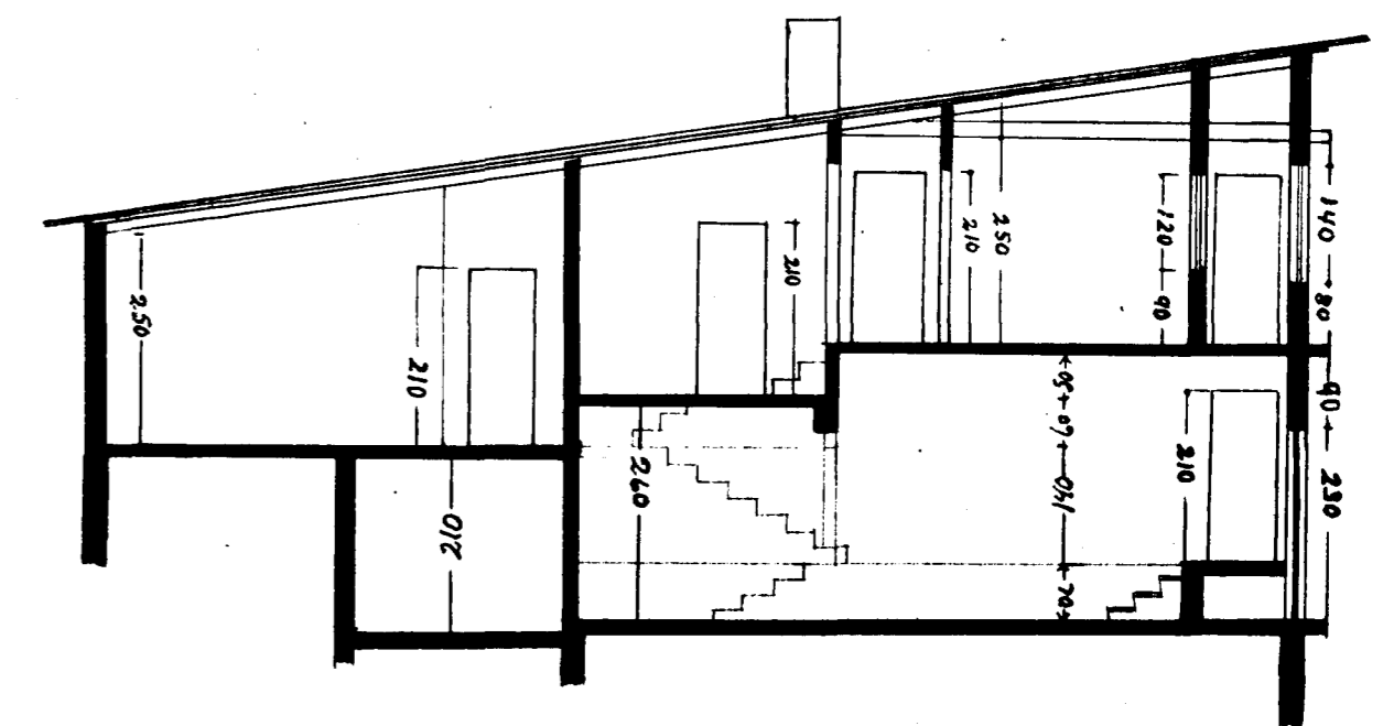
ÞVERSKURÐUR A-A
