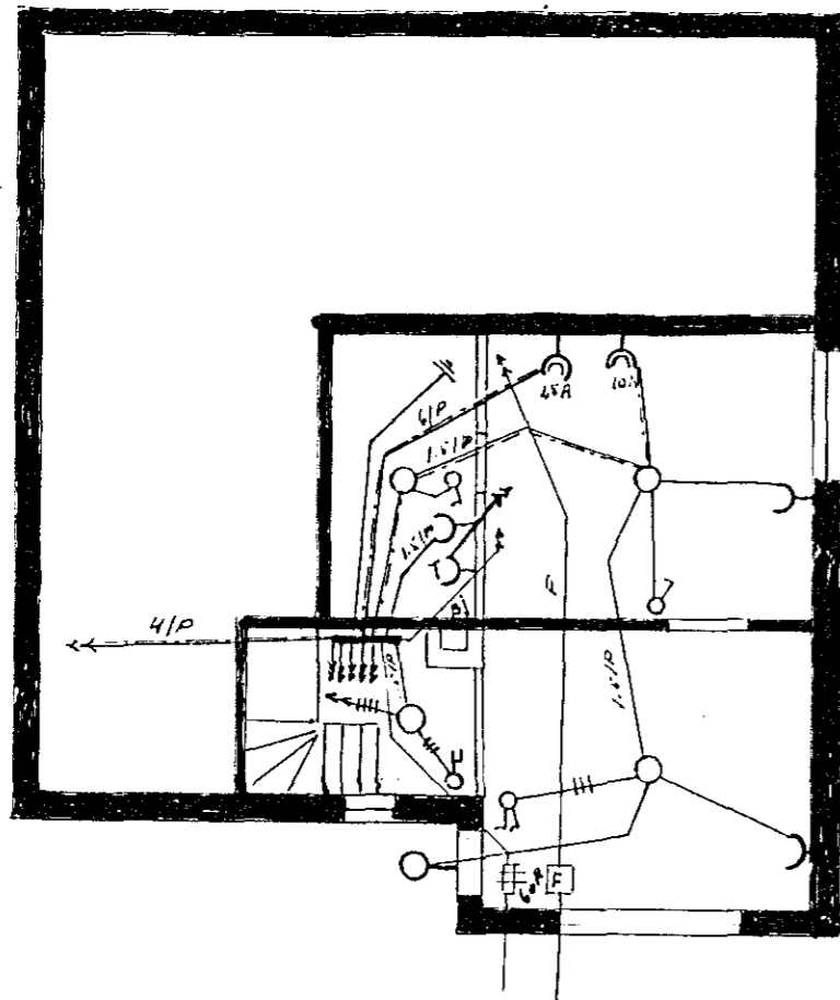
Kjallari
