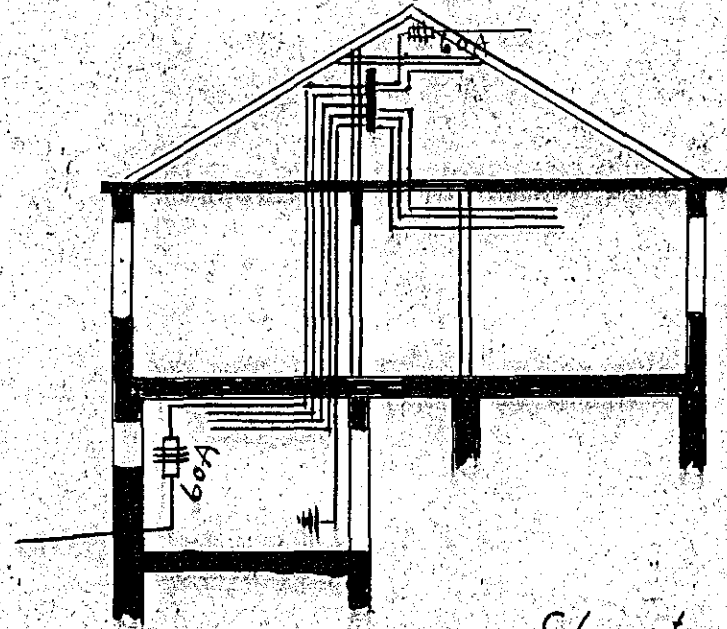
Skurður
