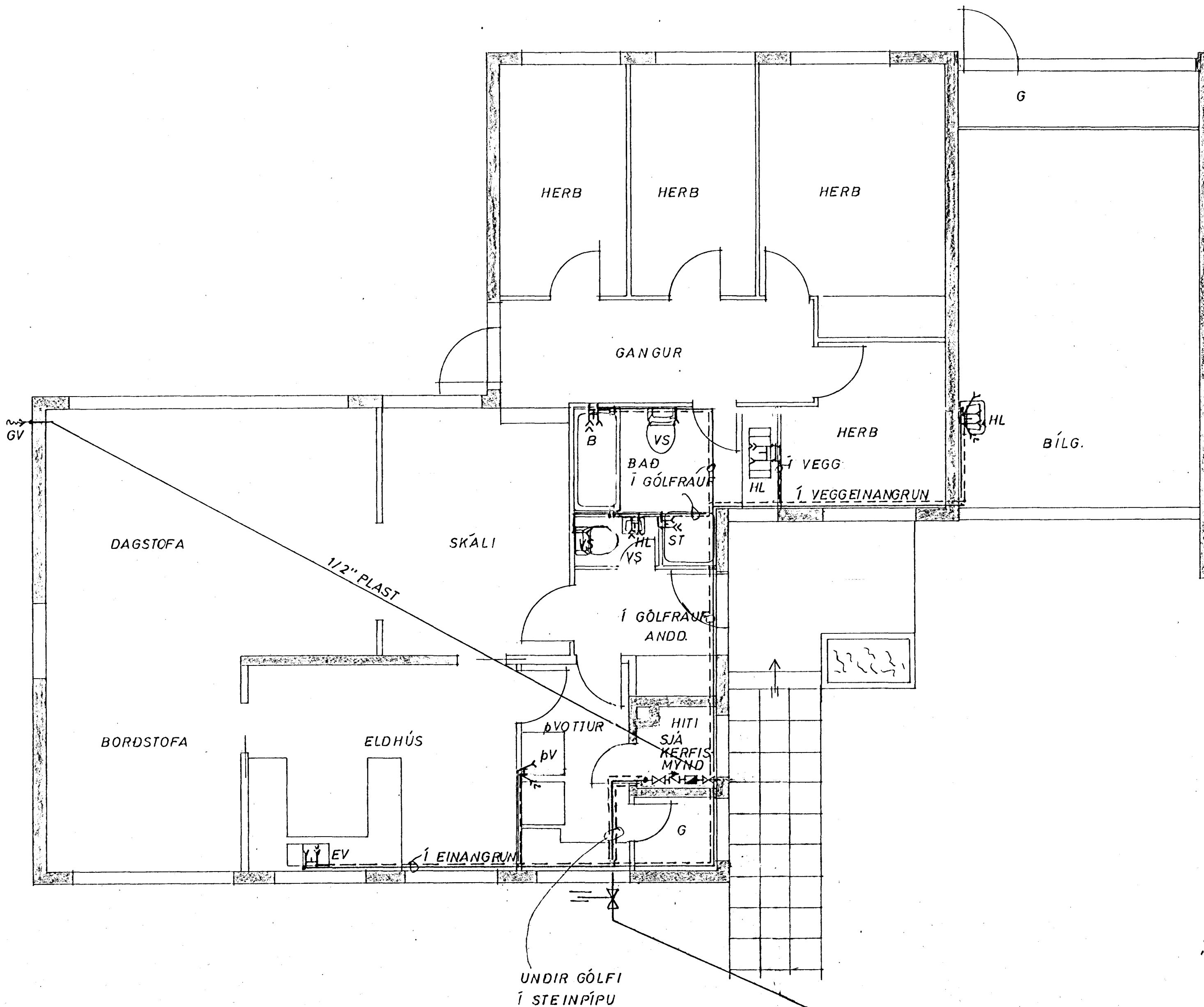
GRUNNMYND 1:50
