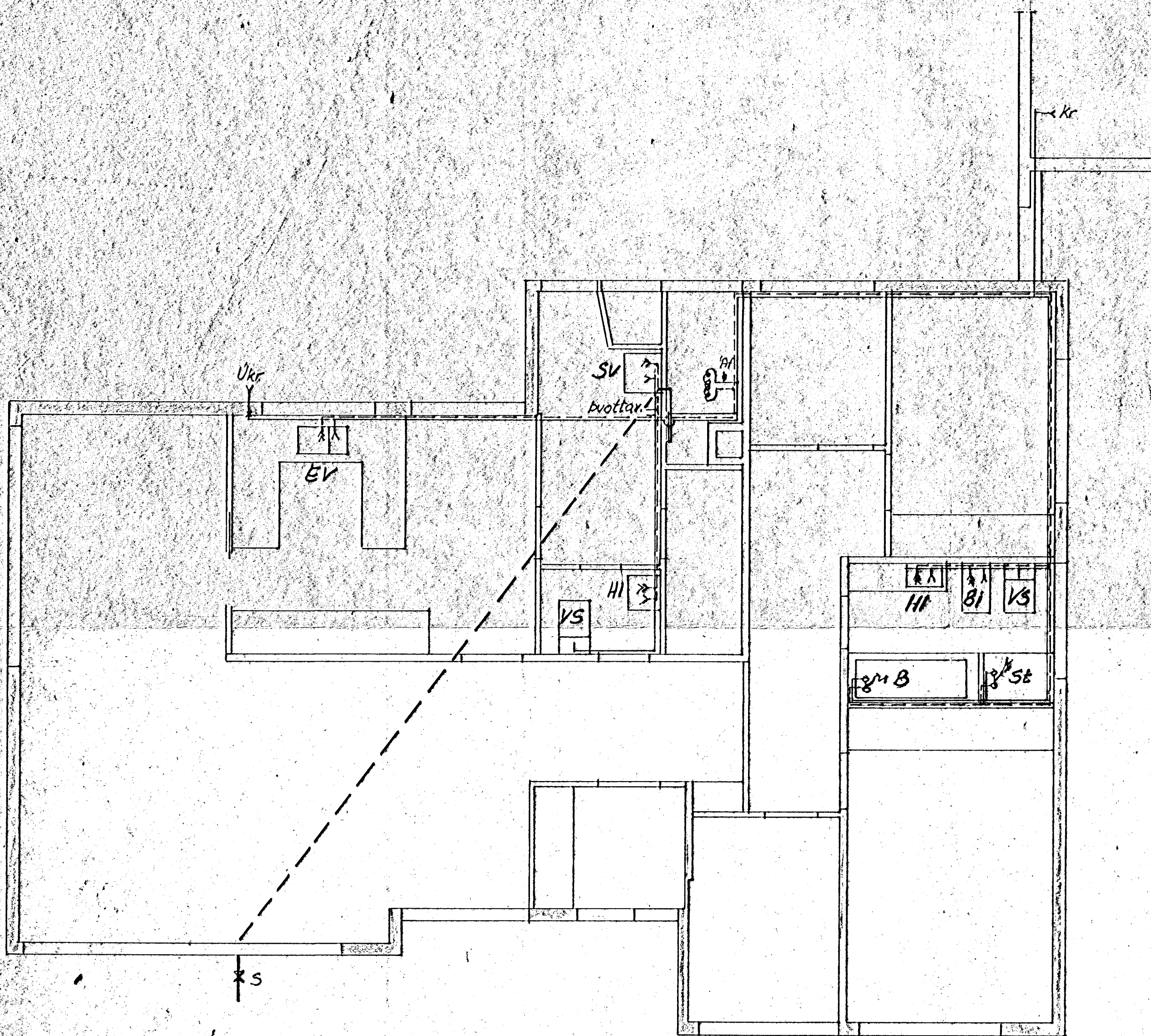
Grunnmynd 1:50
