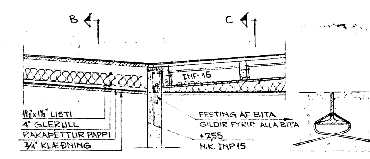
SERTEIKN. I; 1:20
