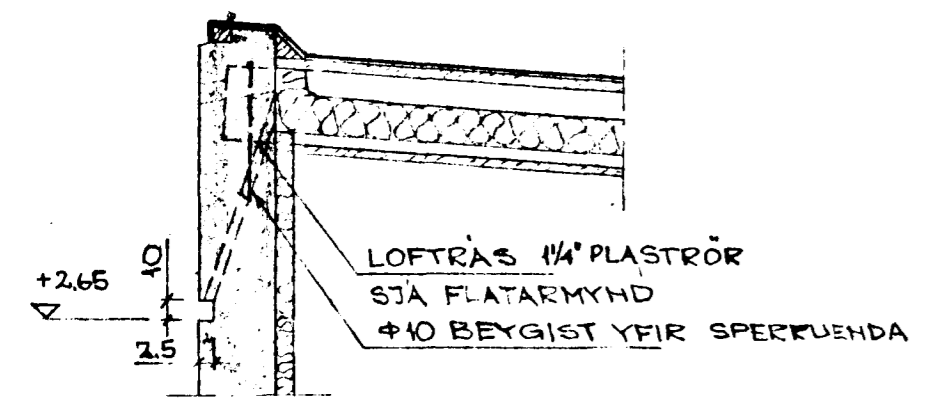
SERTEIKN II; 1:20
