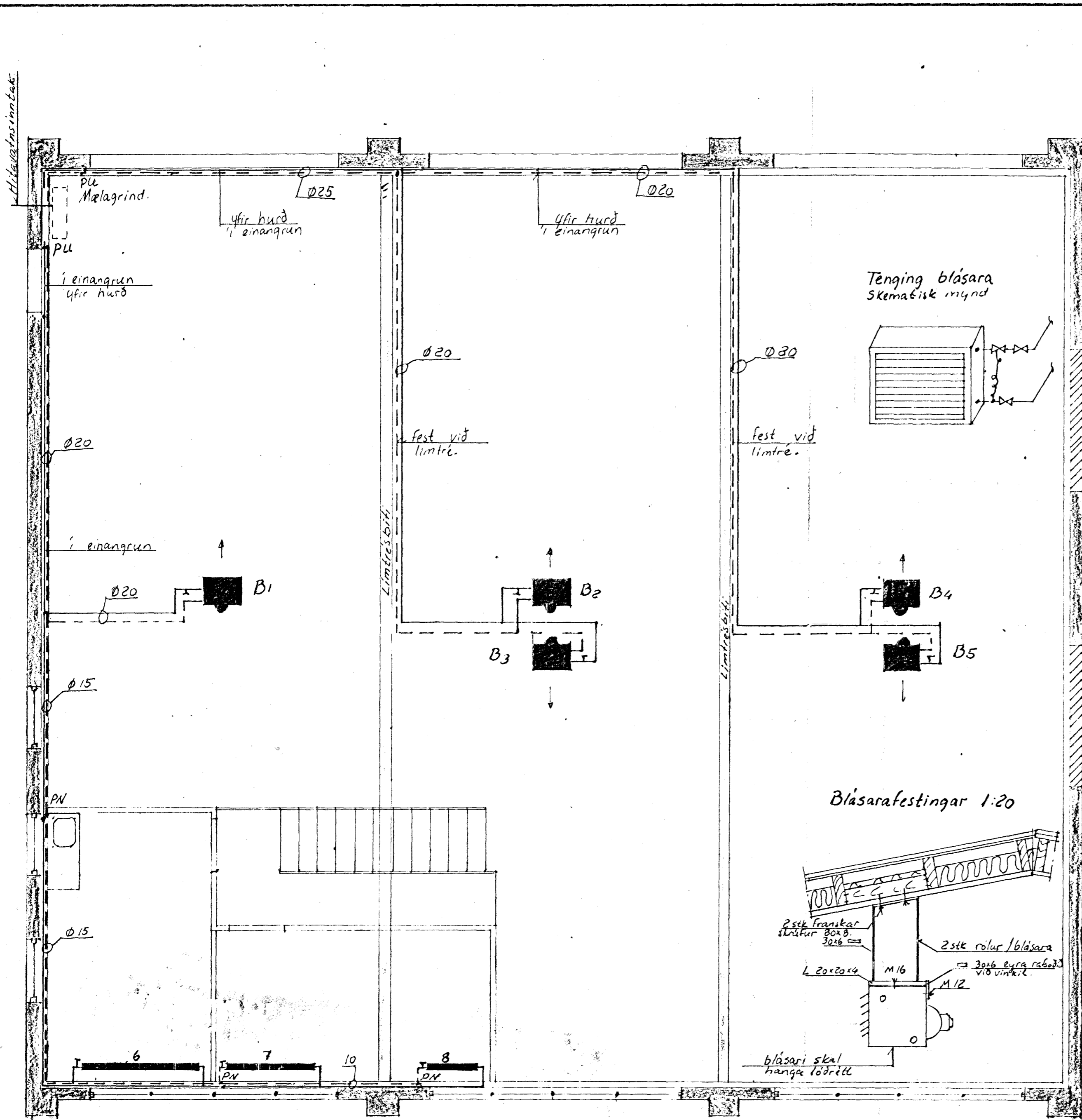
Hitalögn - grunnmynd 1:50 2 hæð og blásara.
