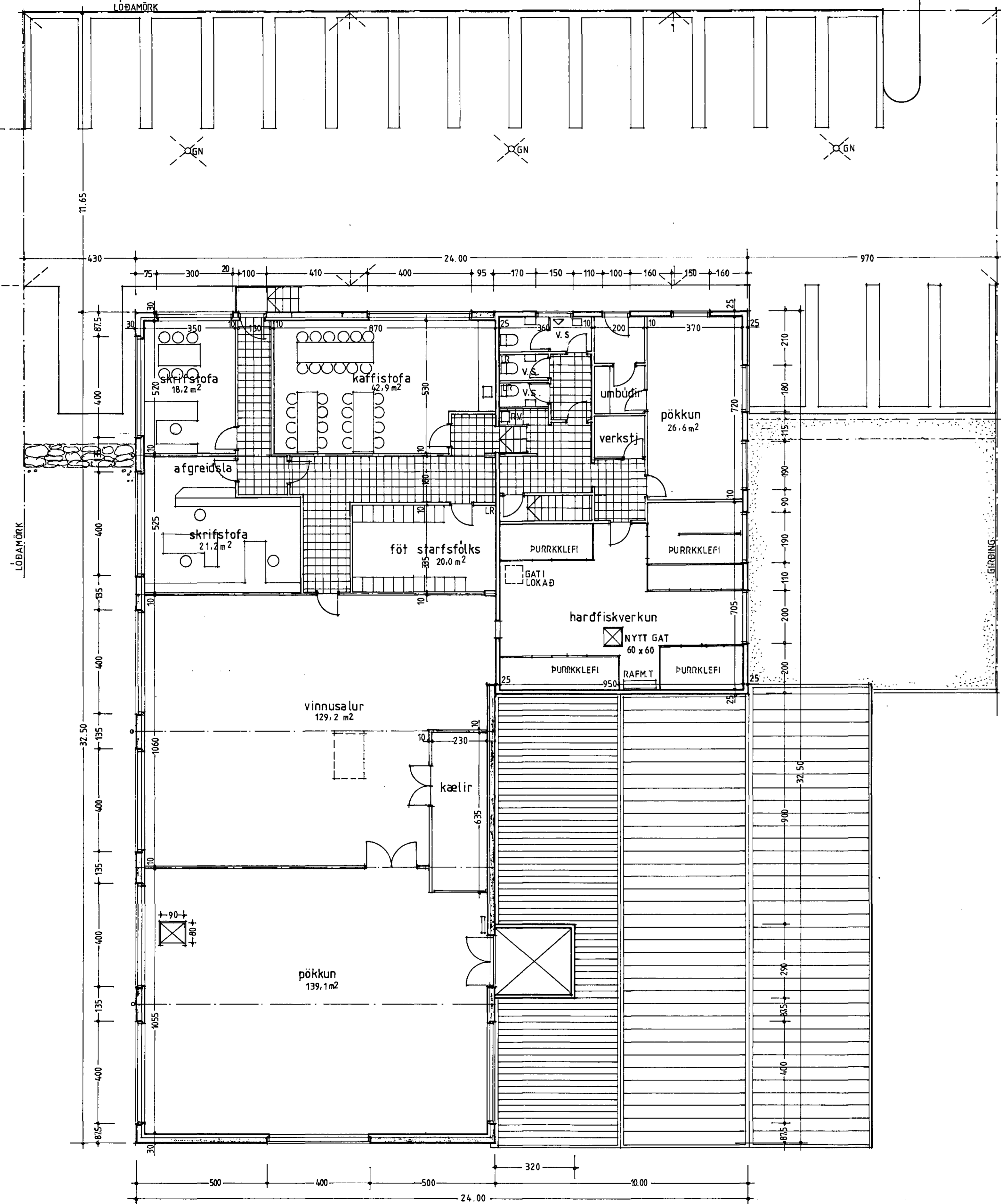
GRUNNMYND EFRI HÆÐ 1:100
