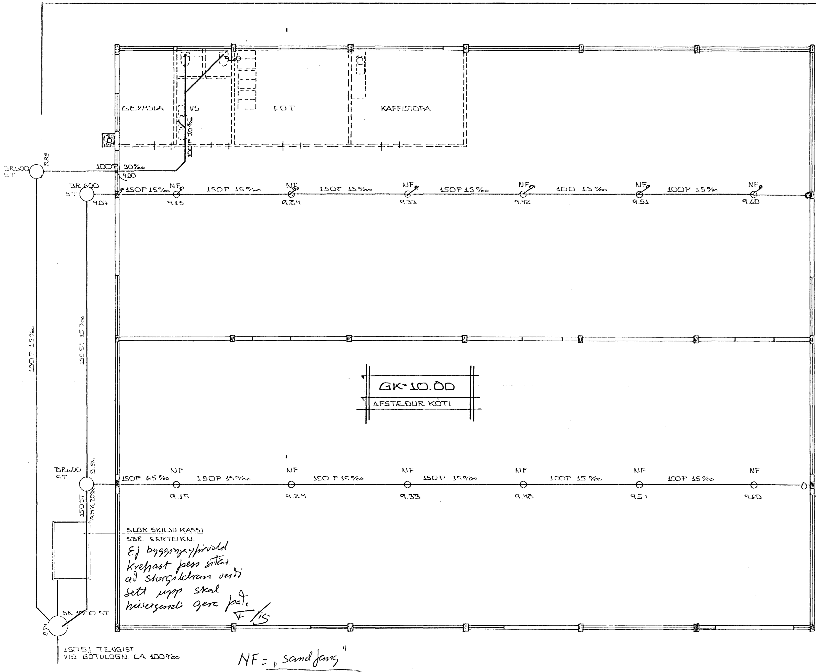
GRUNNMYND 1:100
