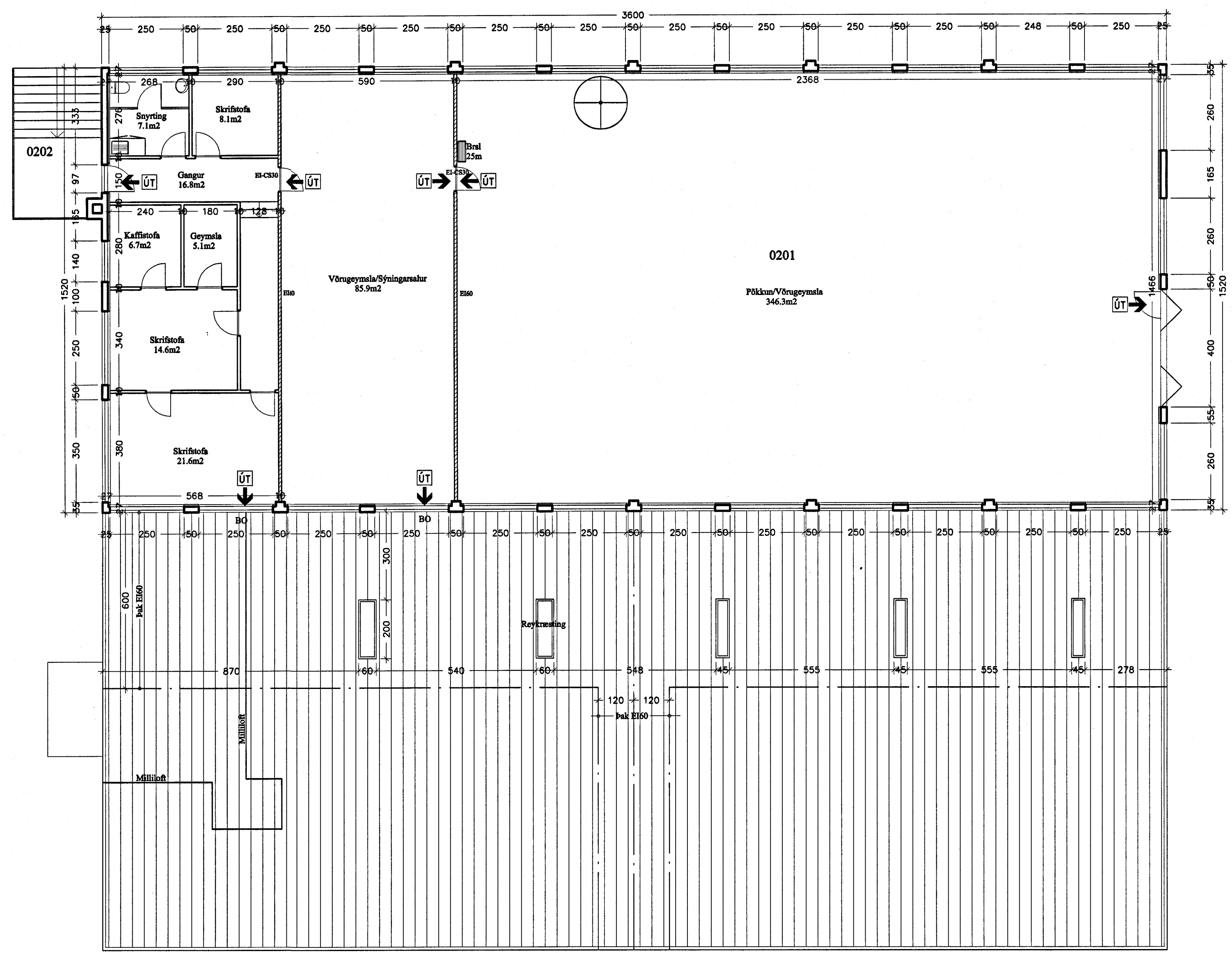
GRUNNMYND 2.HÆÐ 1:100
