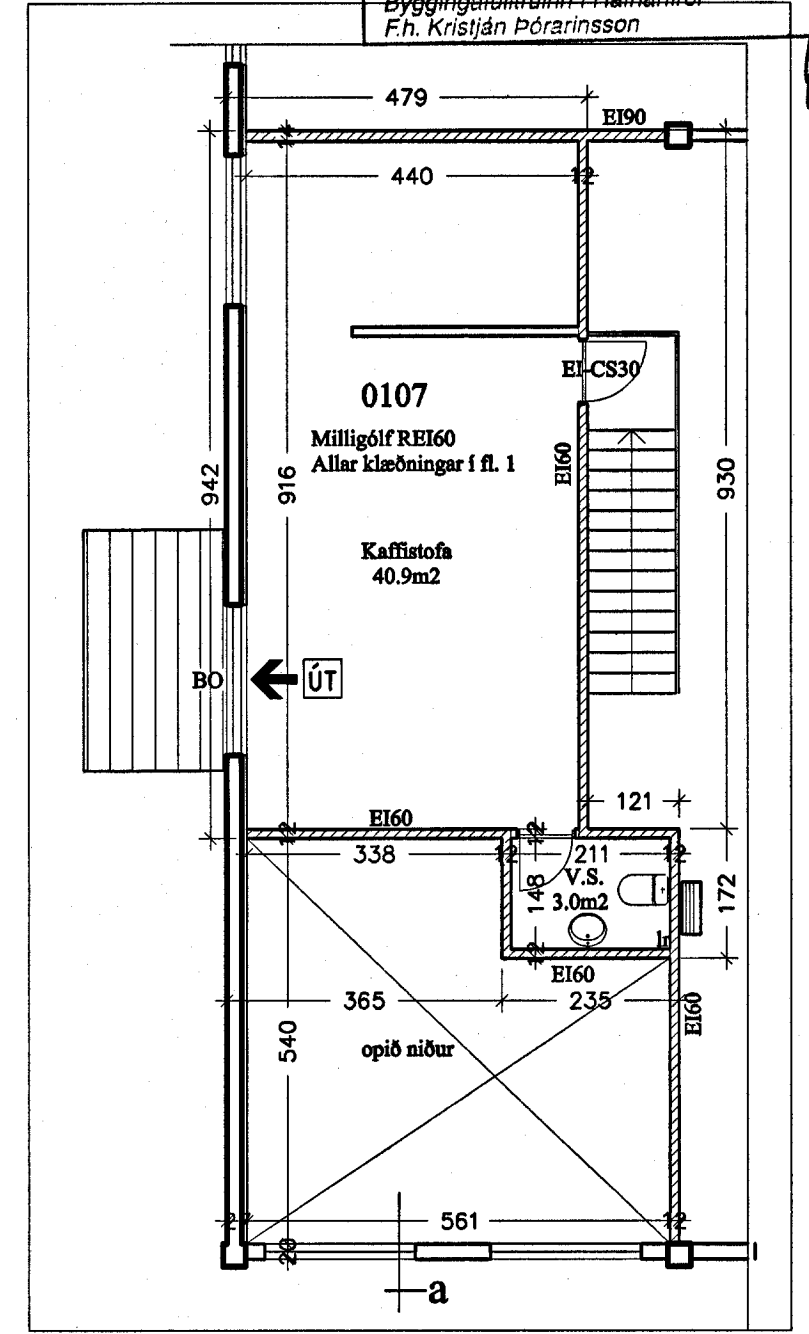
GRUNNMYND MILLILOFT 1:100
