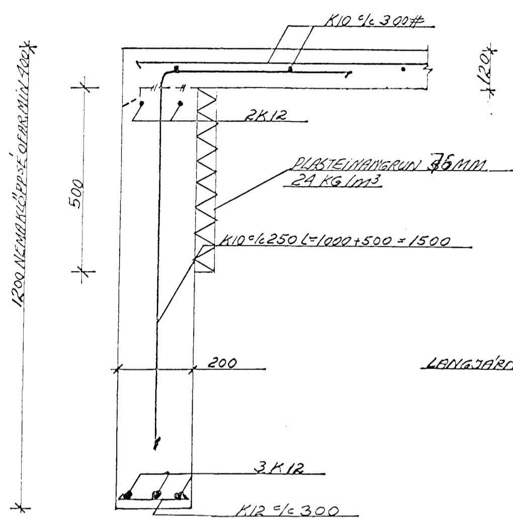
SNÍÐ 2-2 1:10
