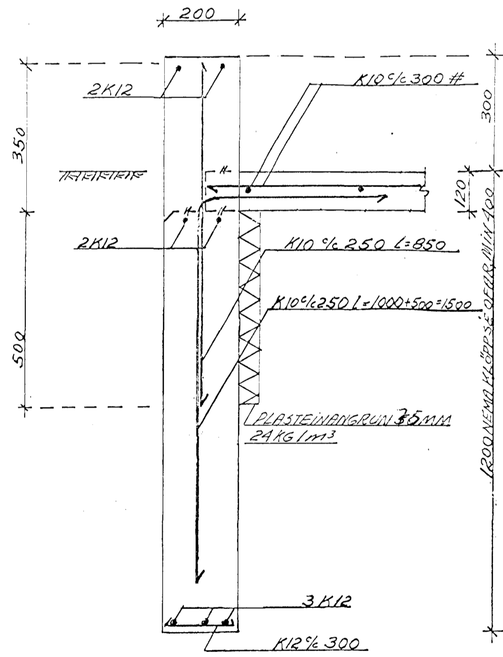
SNÍÐ 1-1 1:10
