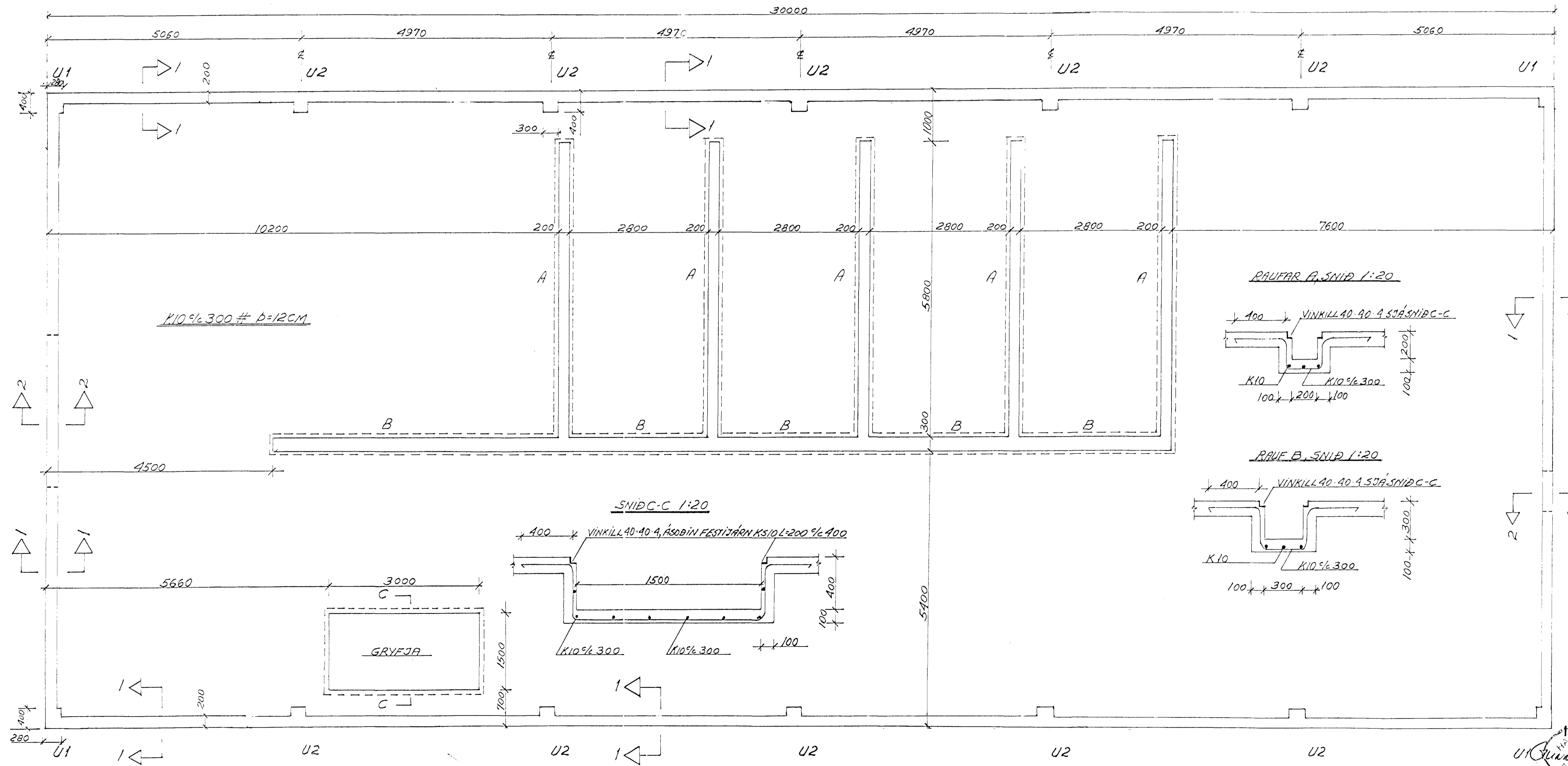
GRUNNMYND 1:50
