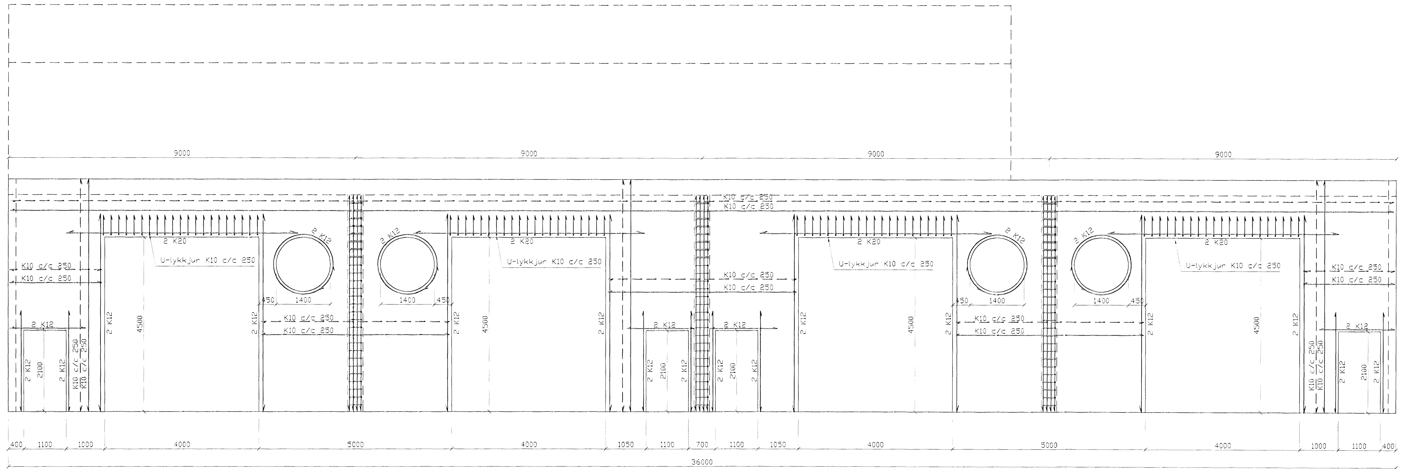
Ásýnd vestur, 1:50
