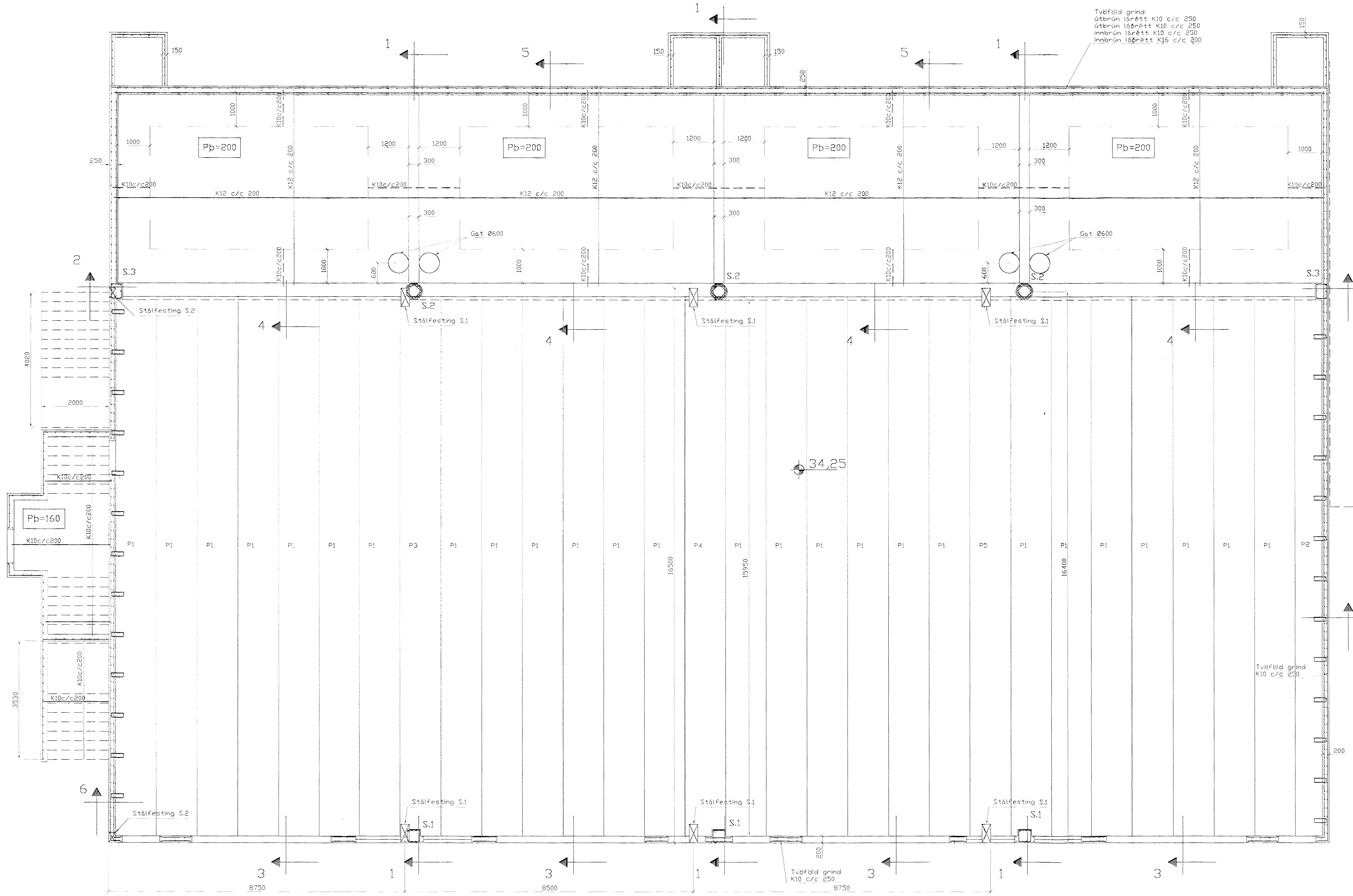
GRUNNMYND 1:50
