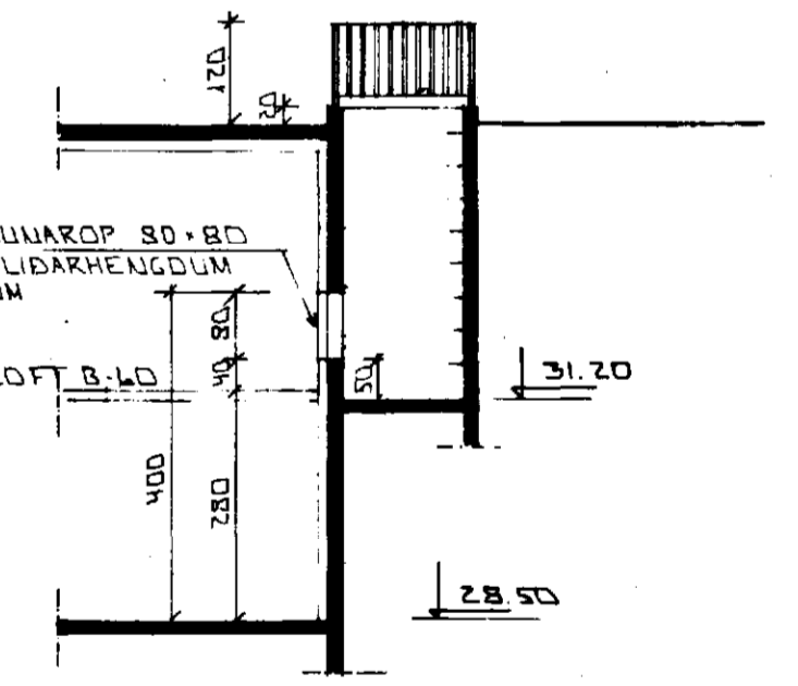
SNID Í BJÖRGUNAROP 1:100
