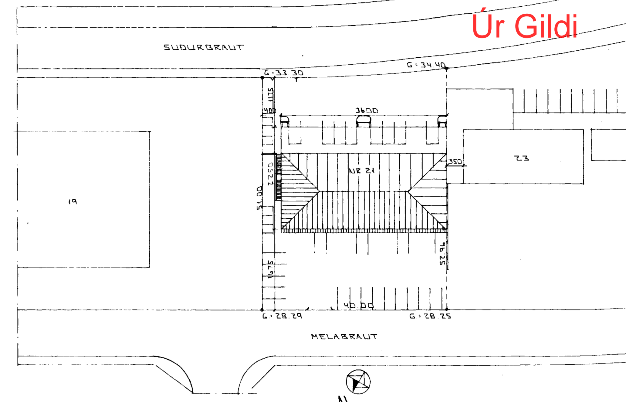
AFSTÖÐUMYND 1:500
