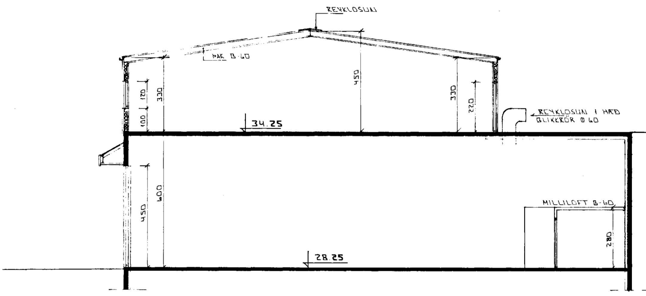
SUÍÐ A-A 1:100
