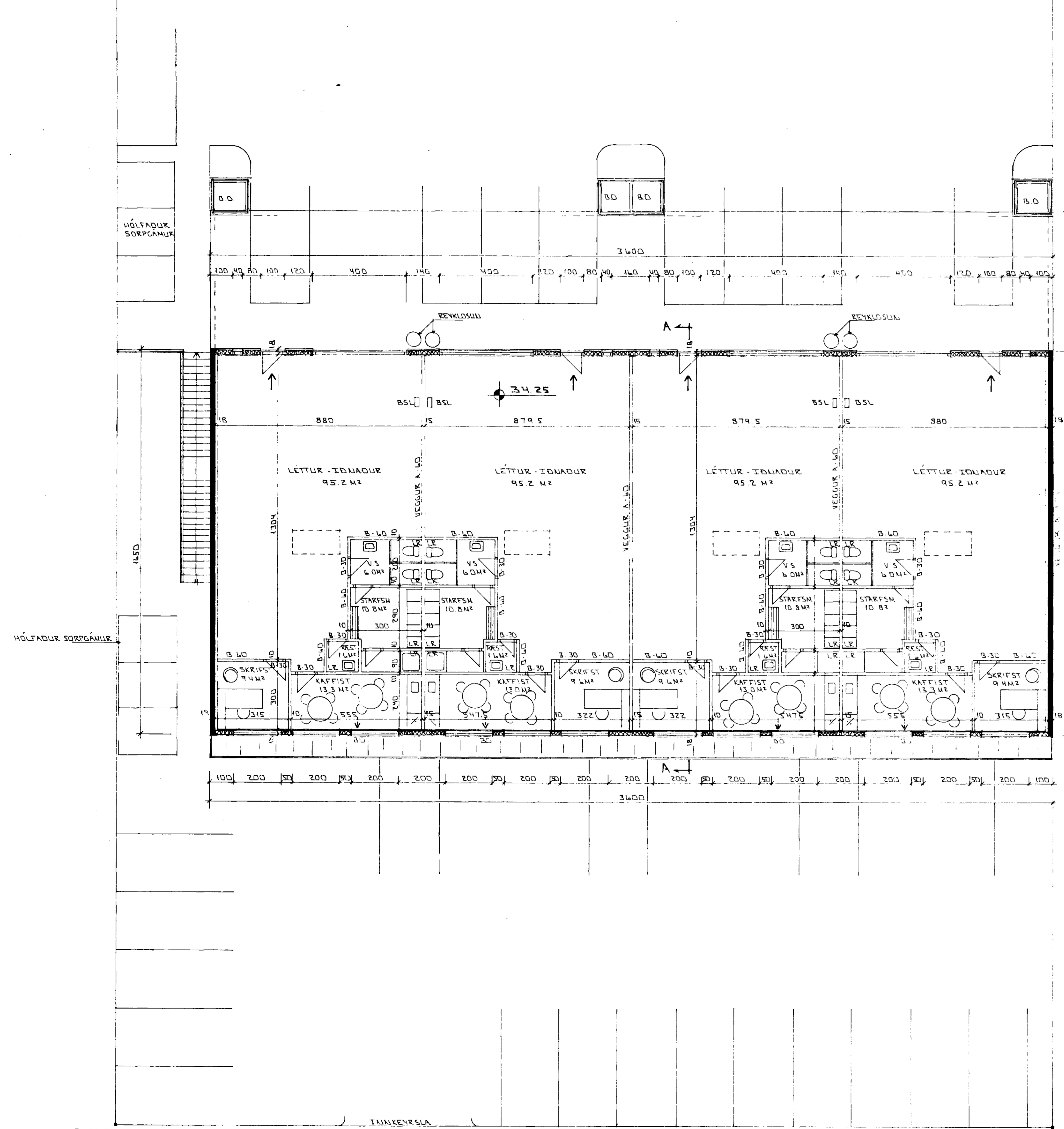
GRUNNMÝND 1:100
