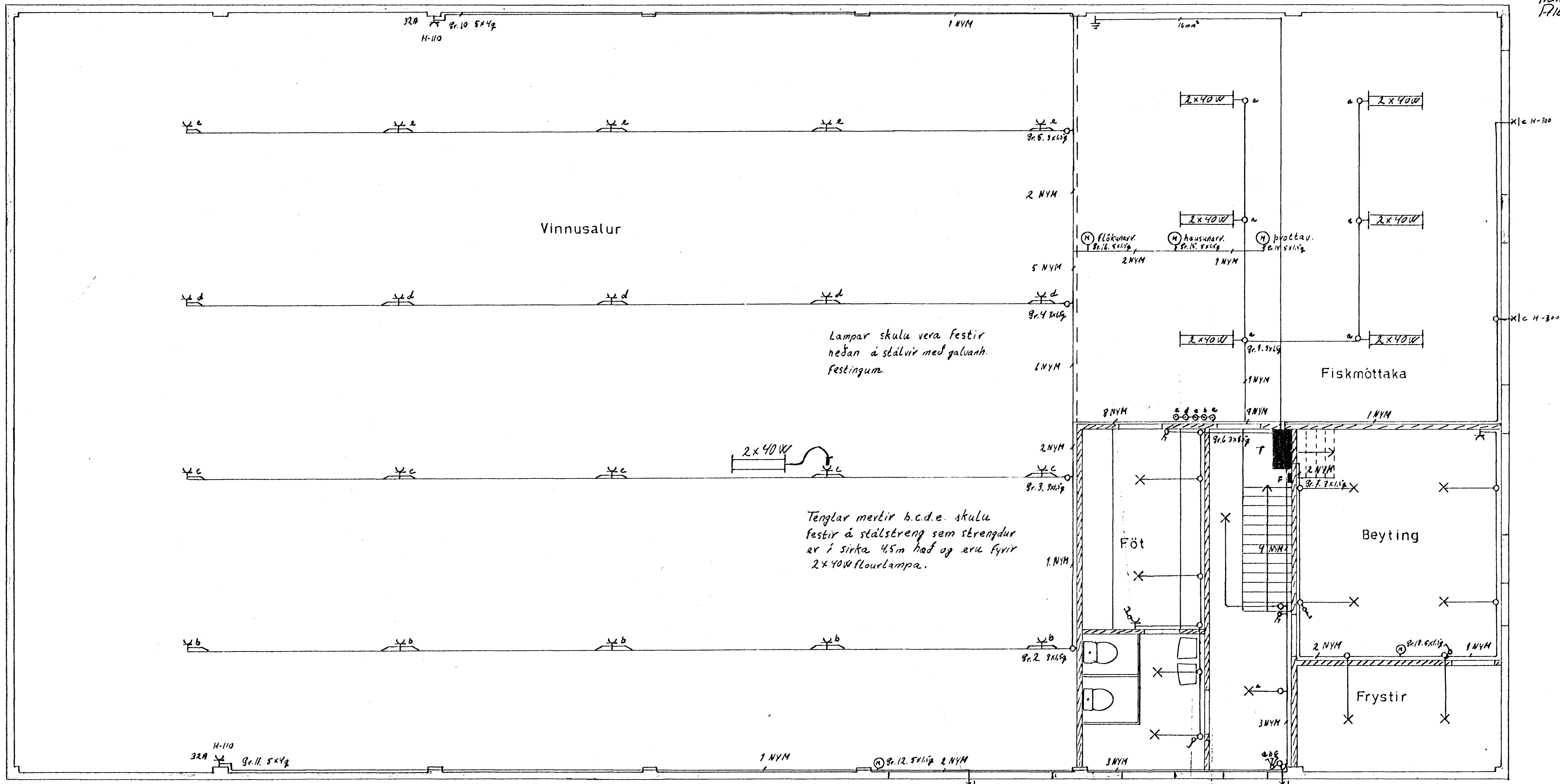
SKÝRINGAR Grunnmynd 1 Hæð 1:50
