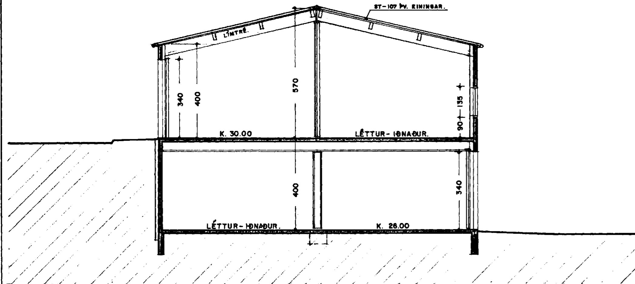
SNEIÐING. 1:100
