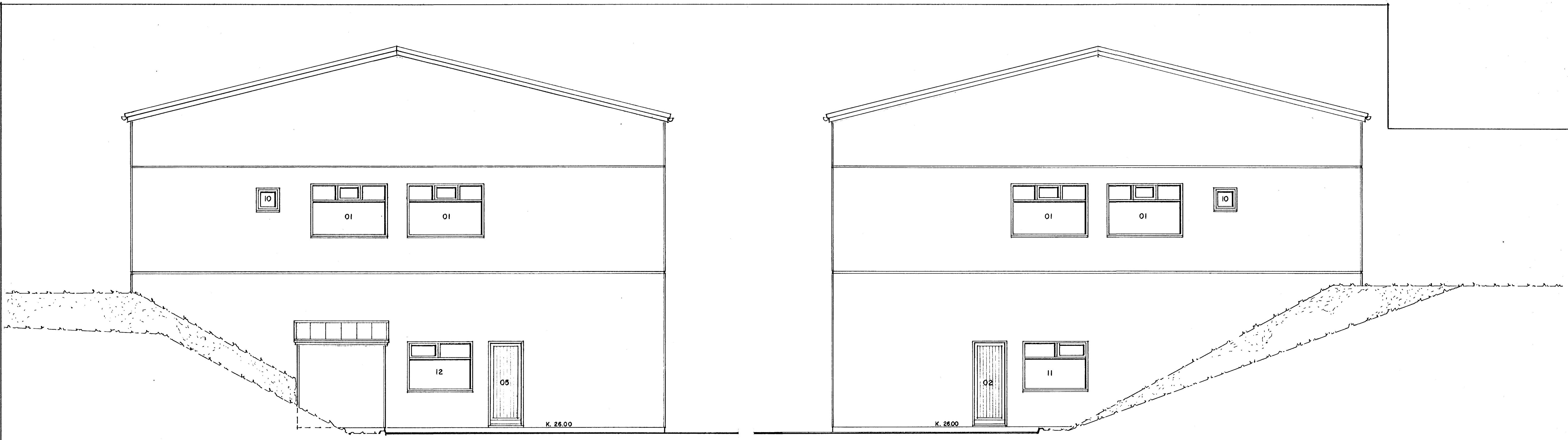
NORÐ - AUSTURHLIÐ. 1:50
