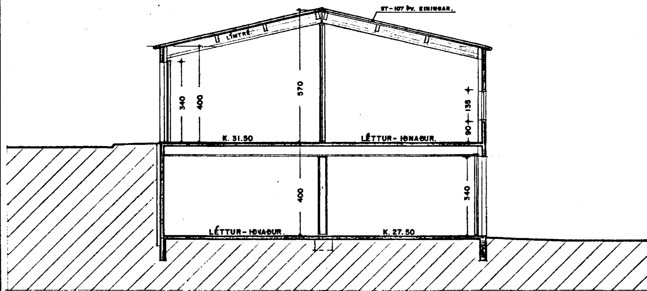
SNEIÐING. 1:100
