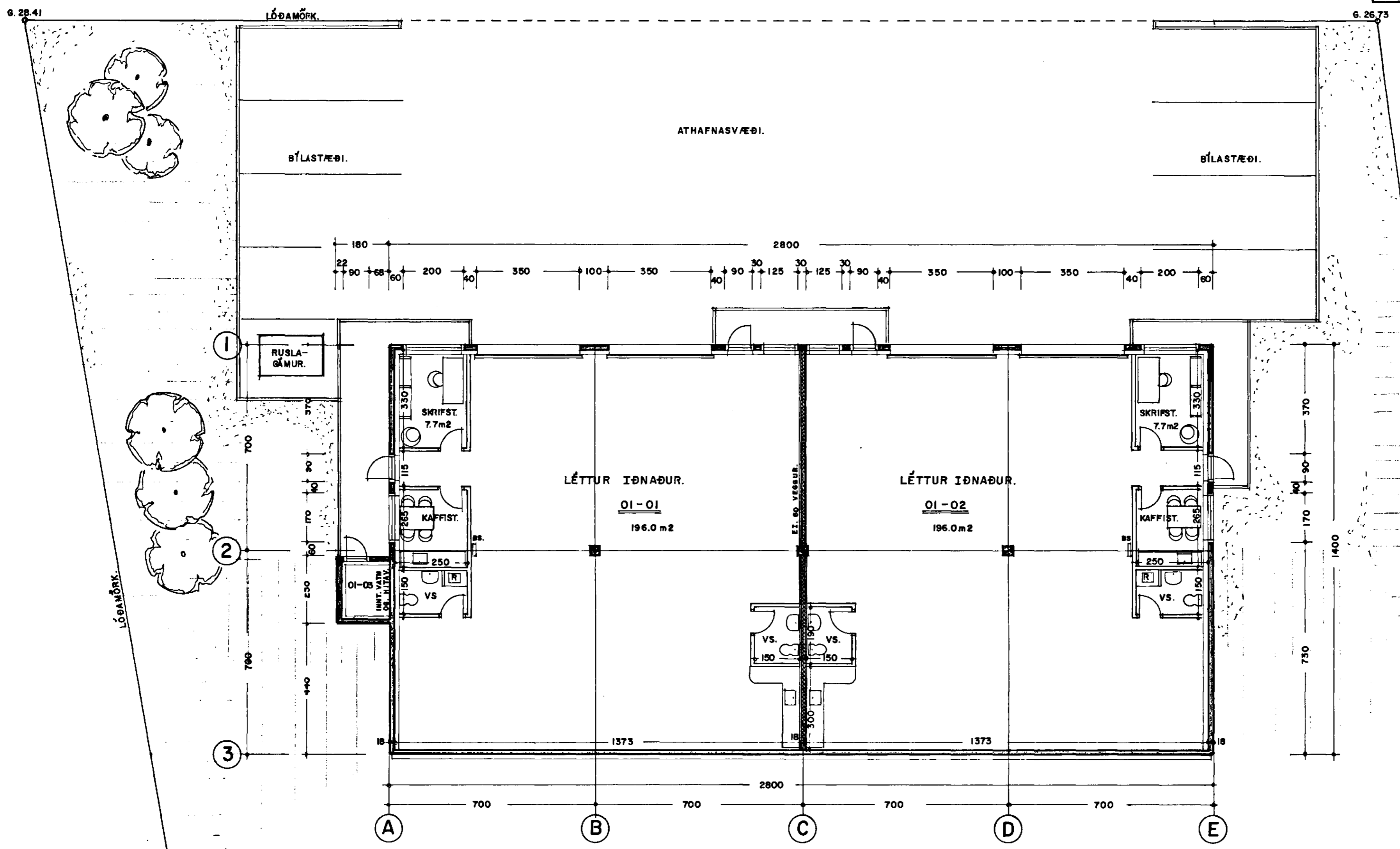
GRUNNMYND I. HÆÐ. 1:100 396.1 m²
