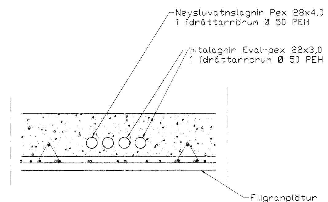
Lagnir í plötu, snið, 1:10
