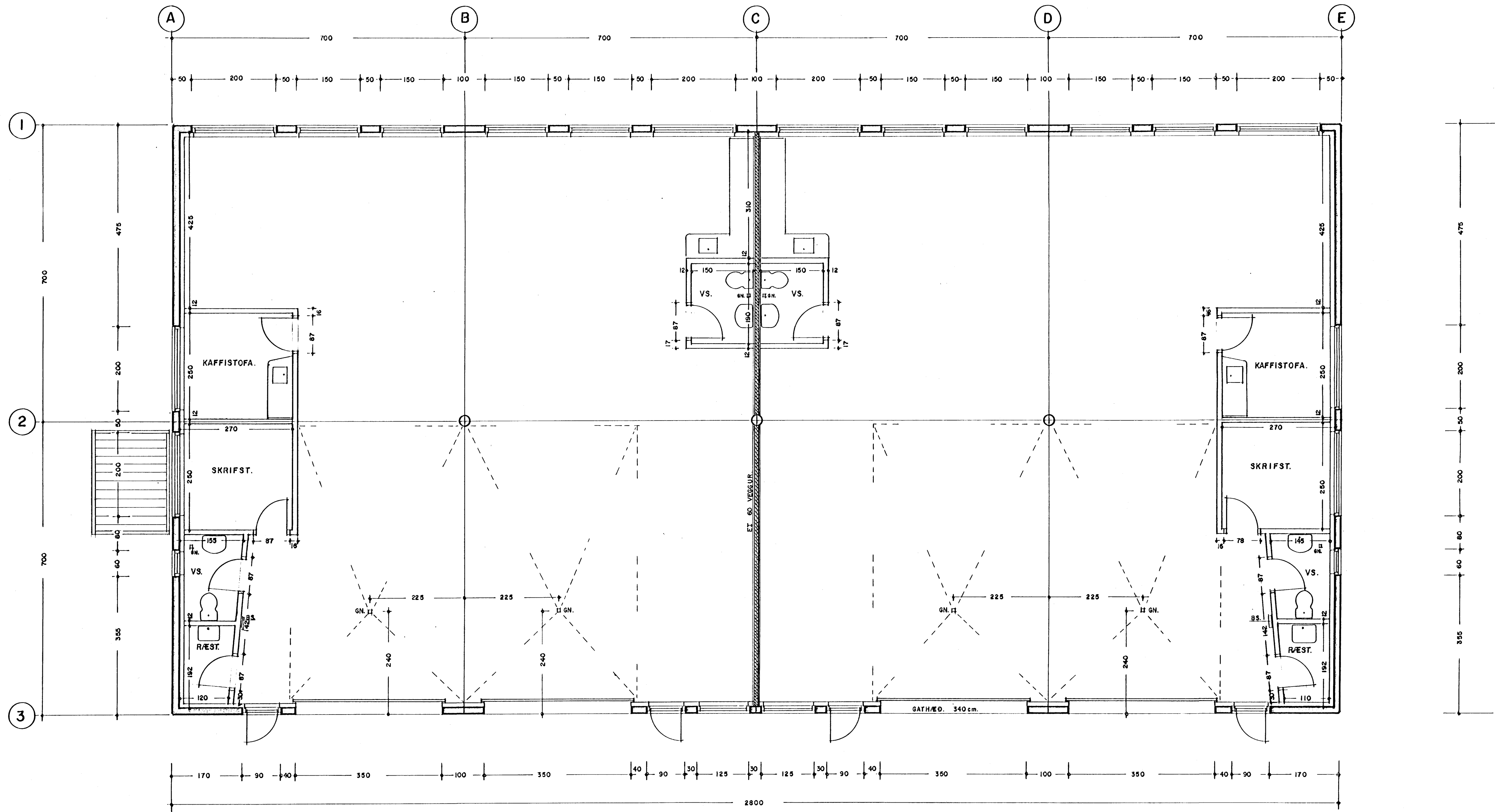
GRUNNMYND 2. HÆÐ. 1:50
