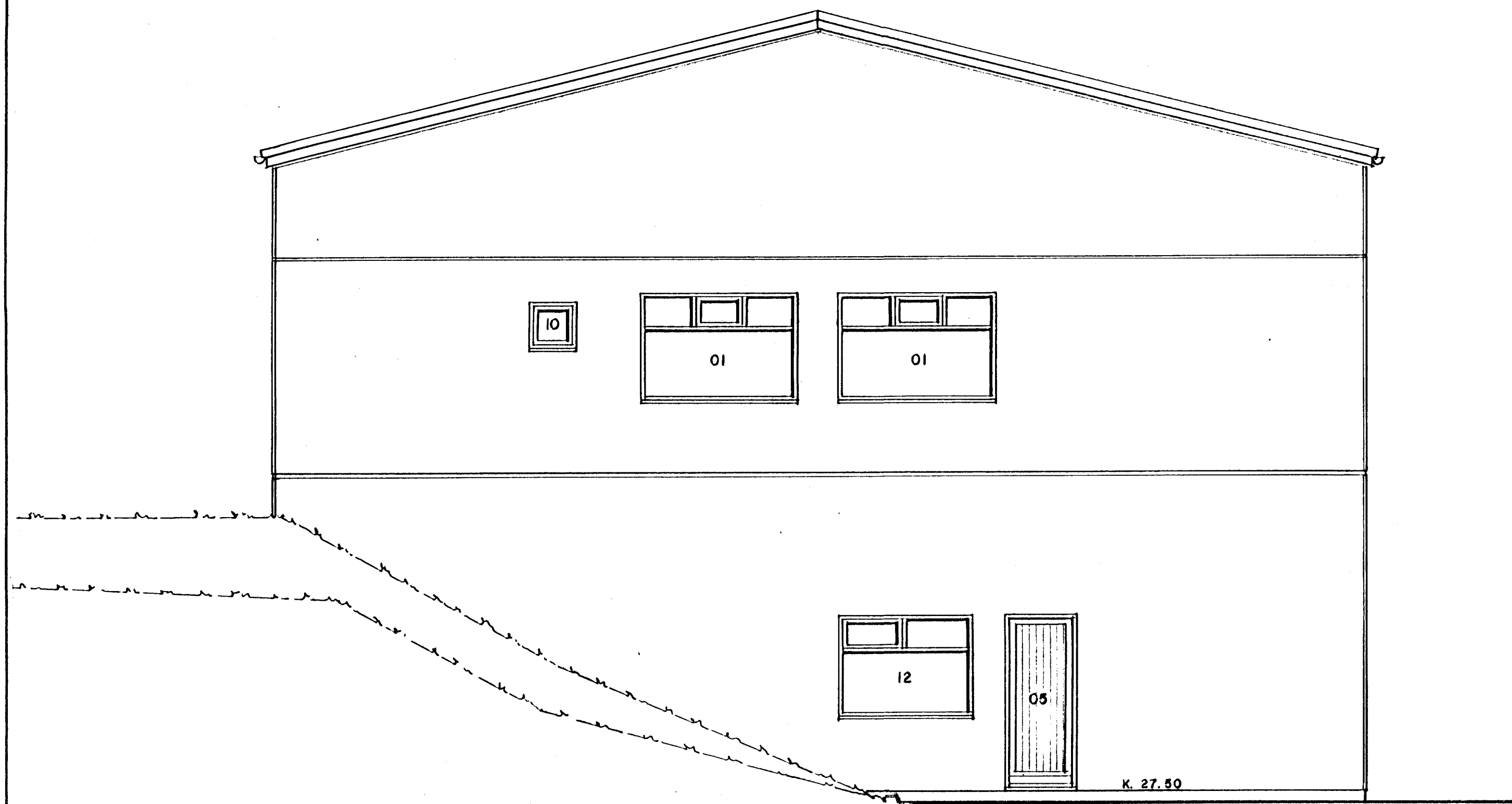
NORÐ - AUSTURHLIÐ. 1:50
