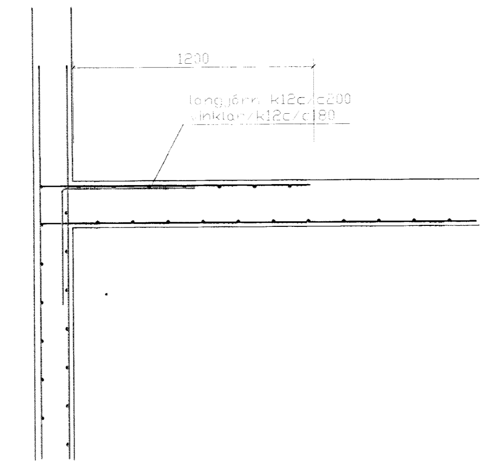
Snið 1 1/20
