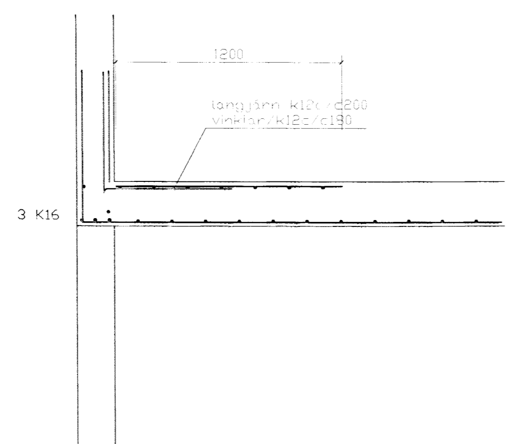
Snið 2 1/20
