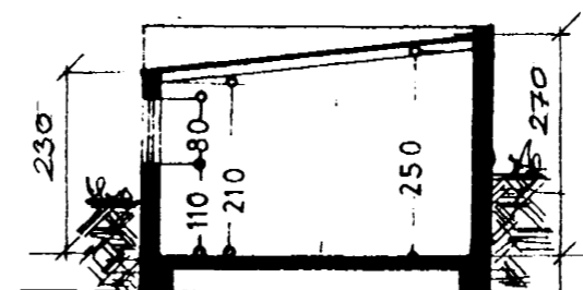
Sníð: A-A
