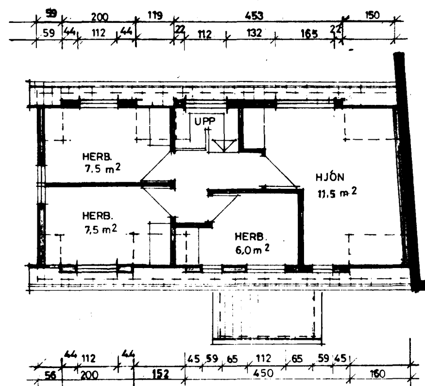
GRUNNMYND RISHÆÐAR 1:100
