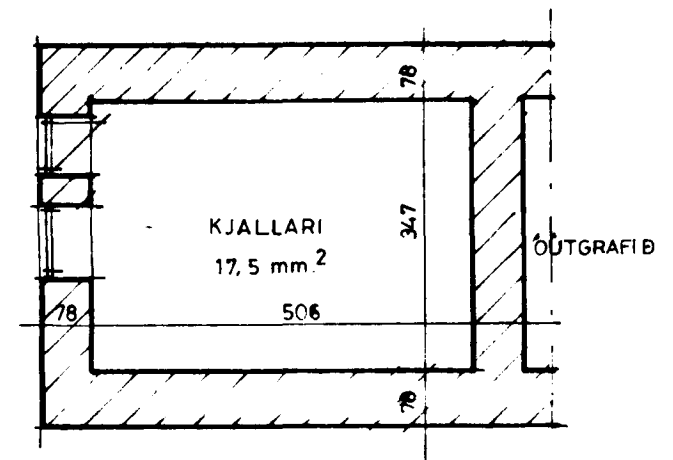
GRUNNMYND KJALLARA
