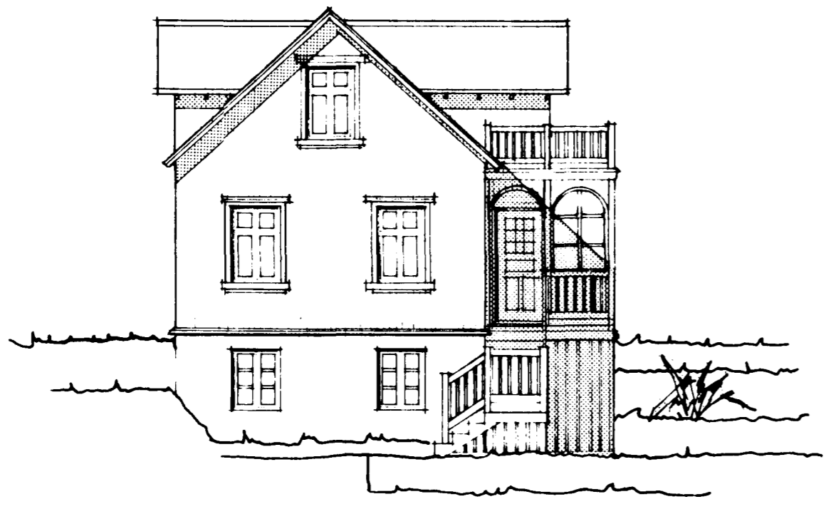
SUÐUR 1:100
