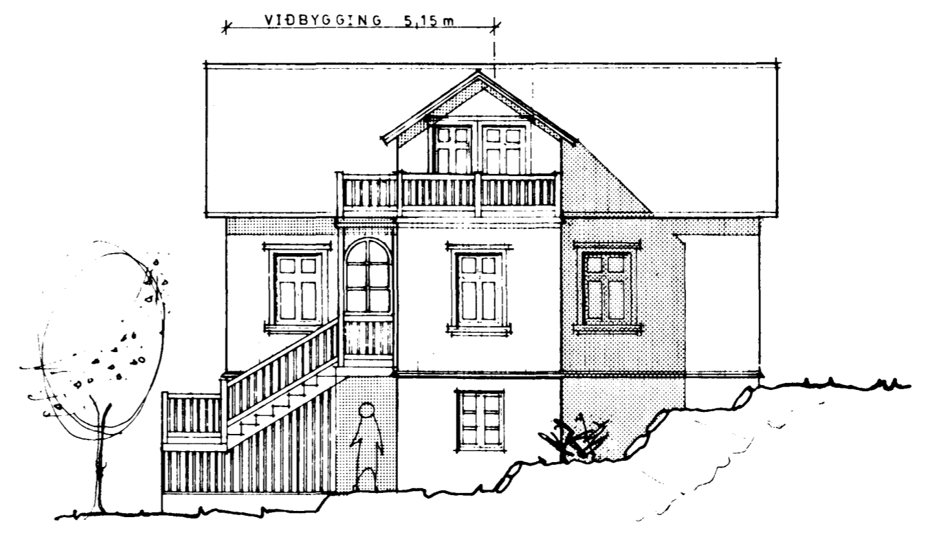
AUSTUR 1:100
