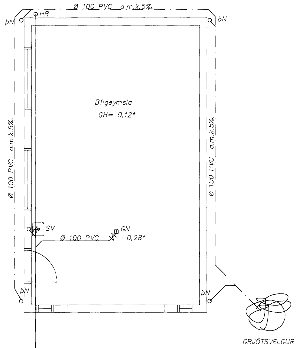
Grundmynd 1:50
