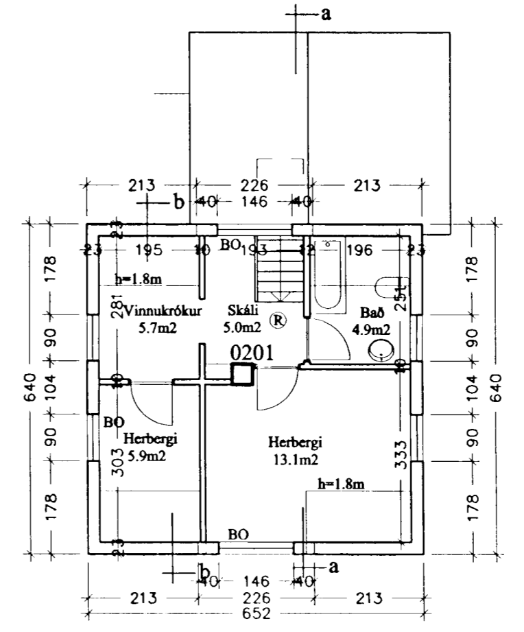
GRUNNMYND RISHÆÐ 1:100
