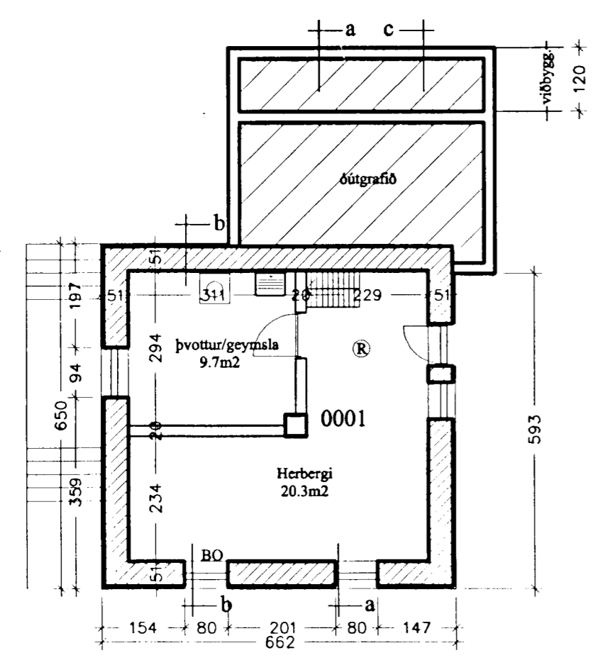
GRUNNMYND KJALLARA 1:100
