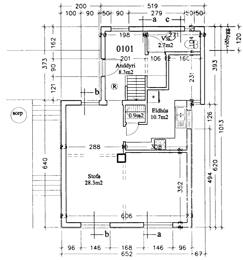
GRUNNMYND 1.HÆÐ 1:100
