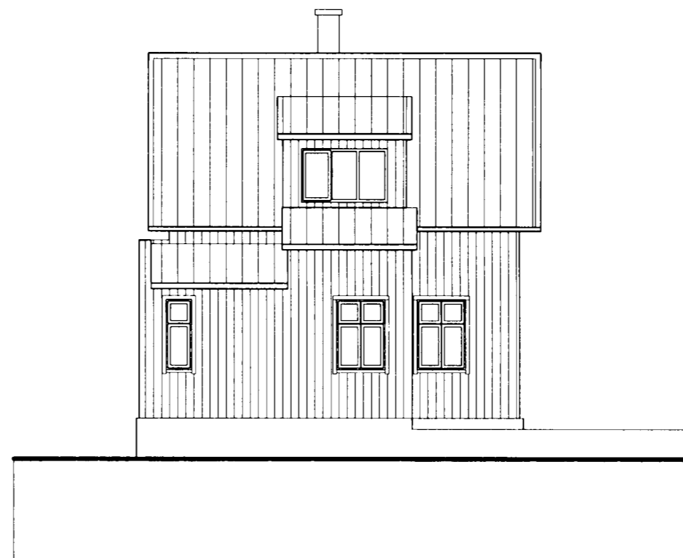
ÚTLIT NORÐUR 1:100
