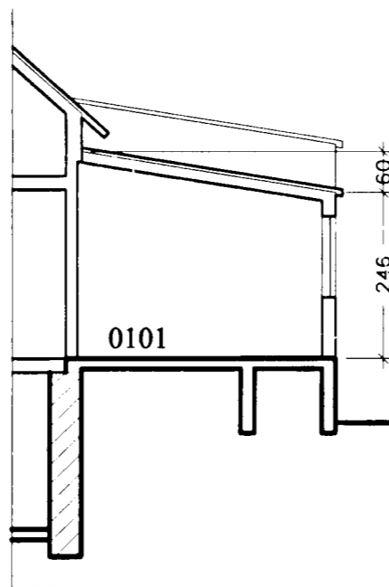
SNEIÐING c 1:100
