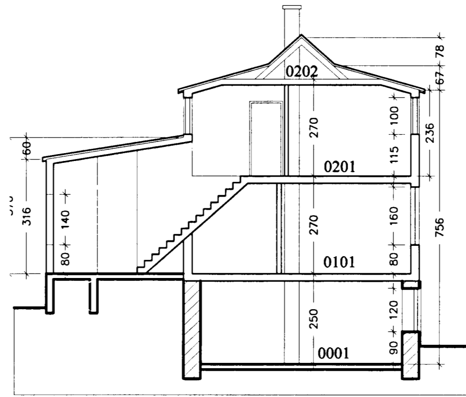
SNEIÐING a-a 1:100
