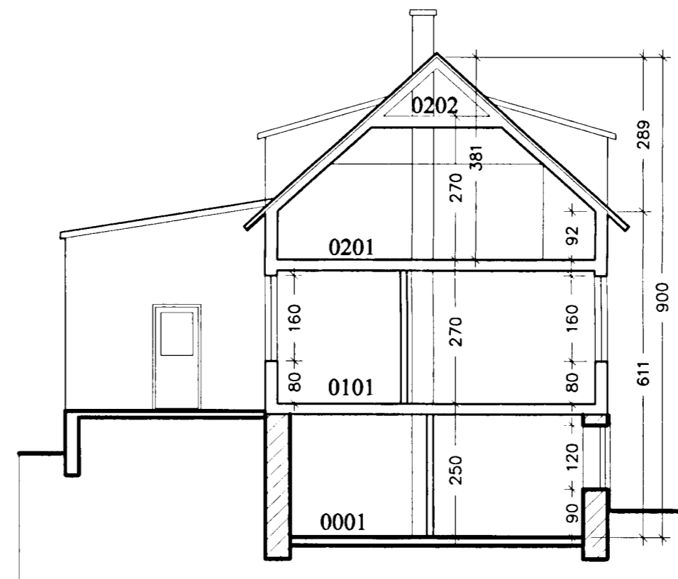
SNEIÐING b-b 1:100
