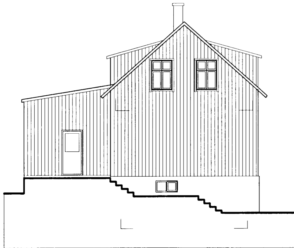
ÚTLIT VESTUR 1:100
