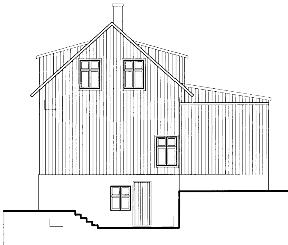
ÚTLIT AUSTUR 1:100
