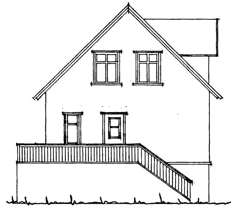
VESTURGAFL 1:100
