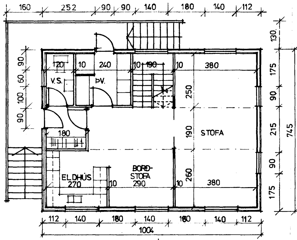
JARÐHÆÐ 1:100
