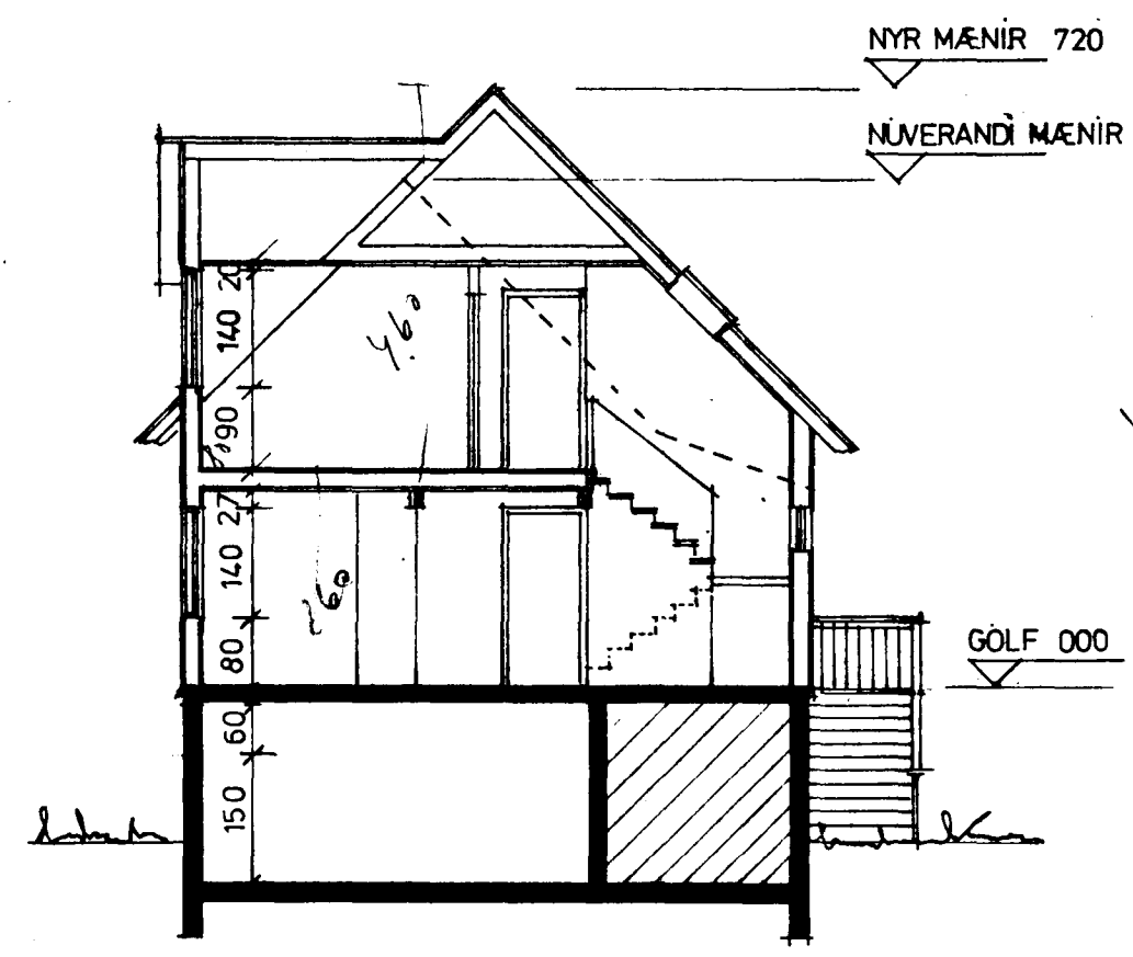
ÞVERSNIÐ A-A 1:100
