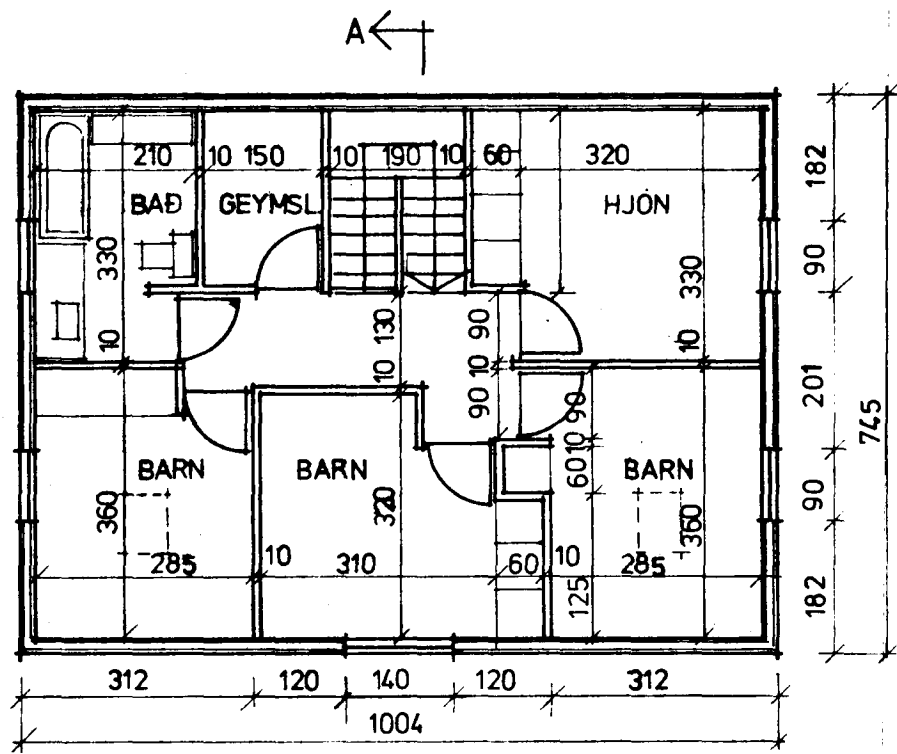
RISHÆÐ 1:100
