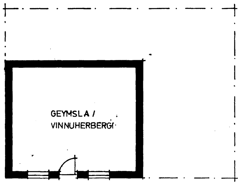
KJALLARI 1:100
