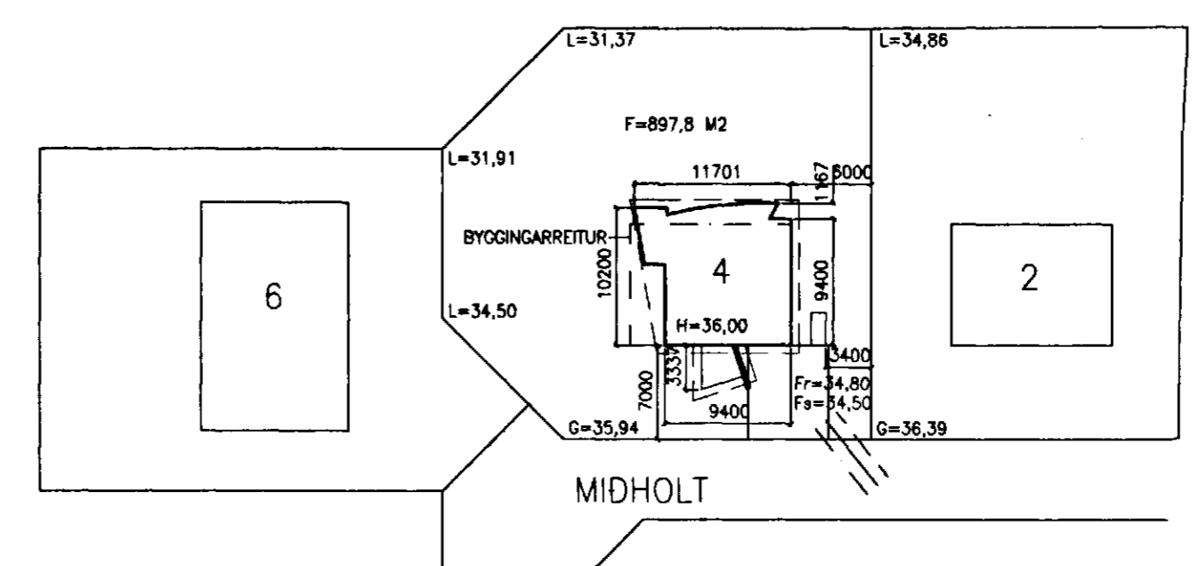
AFSTÖDUMYND MKV. 1:500
