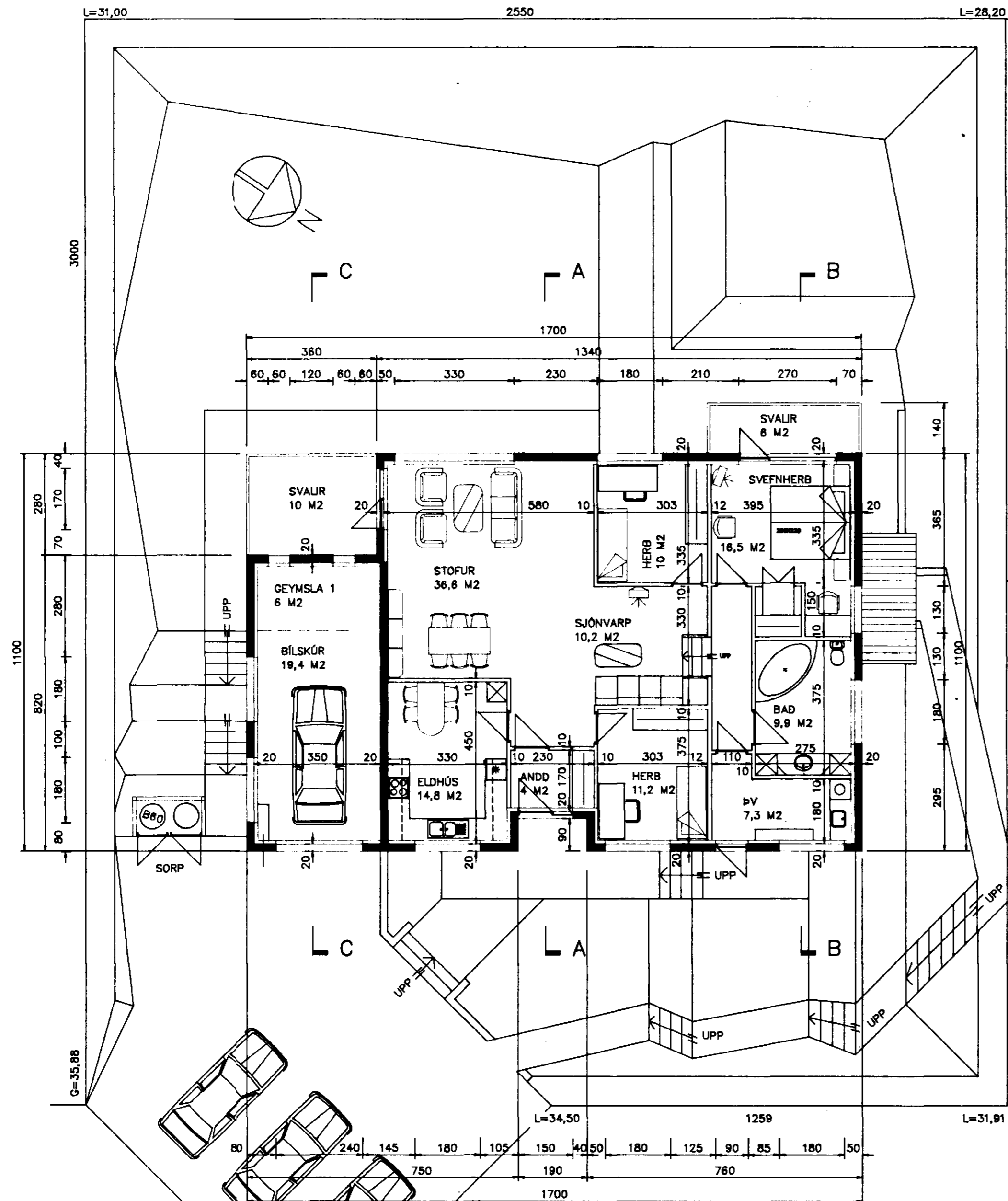
GRUNNMYND EFRI HÆÐAR, M=1:100
