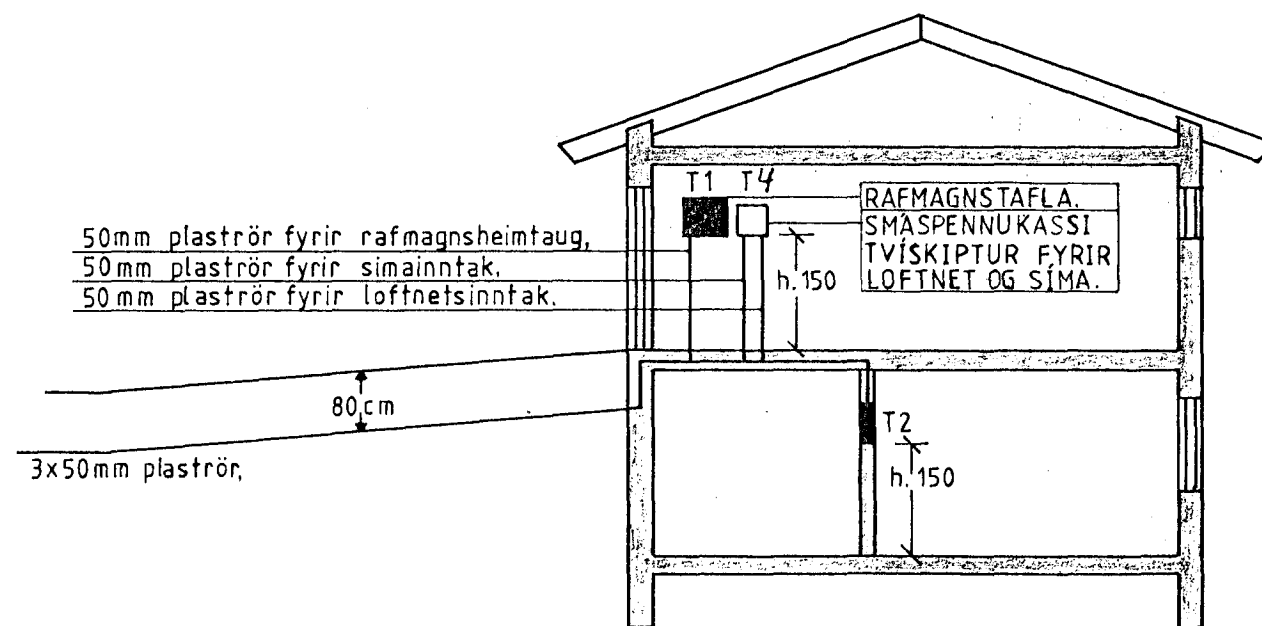
SNÍÐ. A-A. MKV. 1:100.
